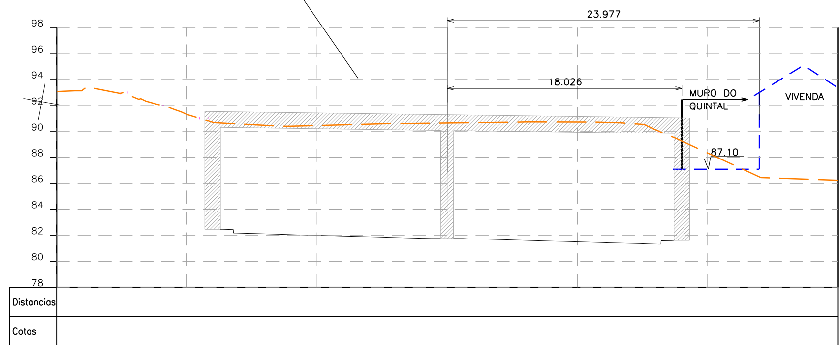
PERFIL TRANSVERSAL AO km 1+115
