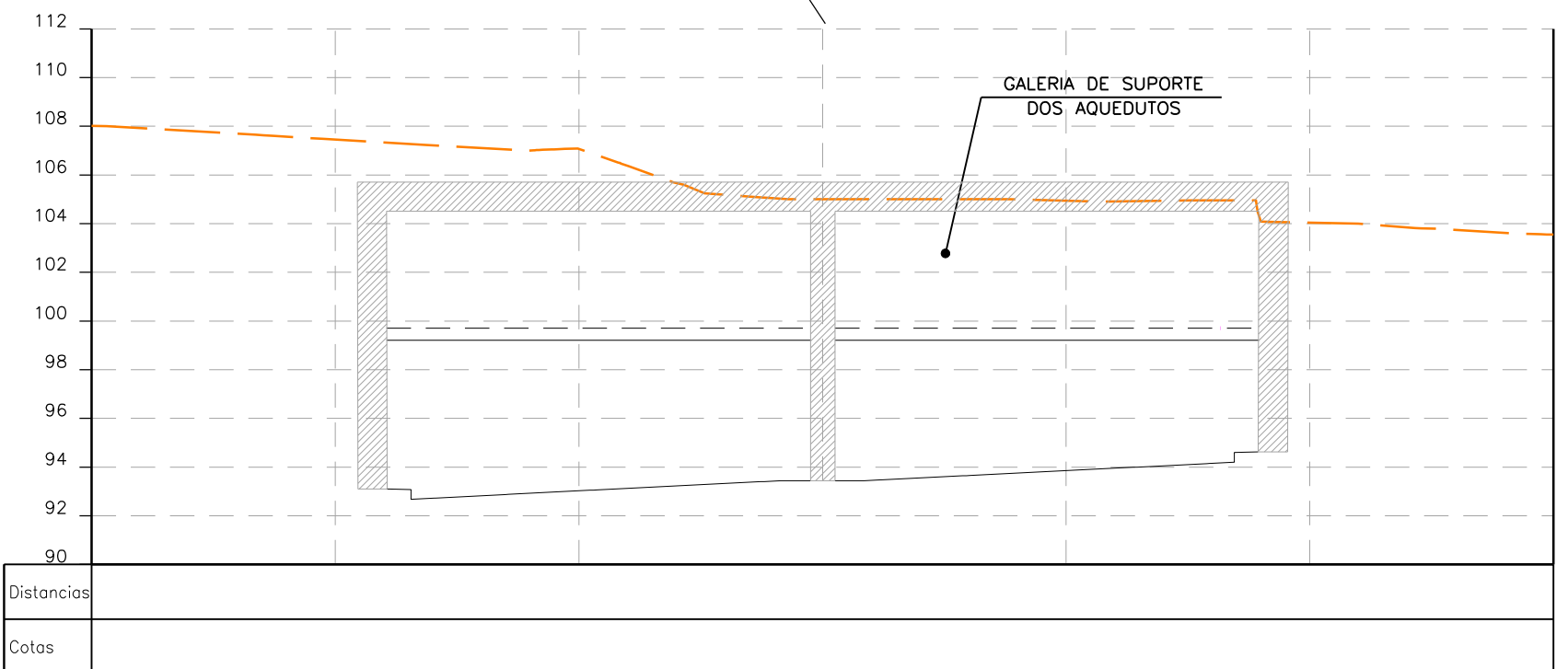
PERFIL TRANSVERSAL AO km 0+708,7
