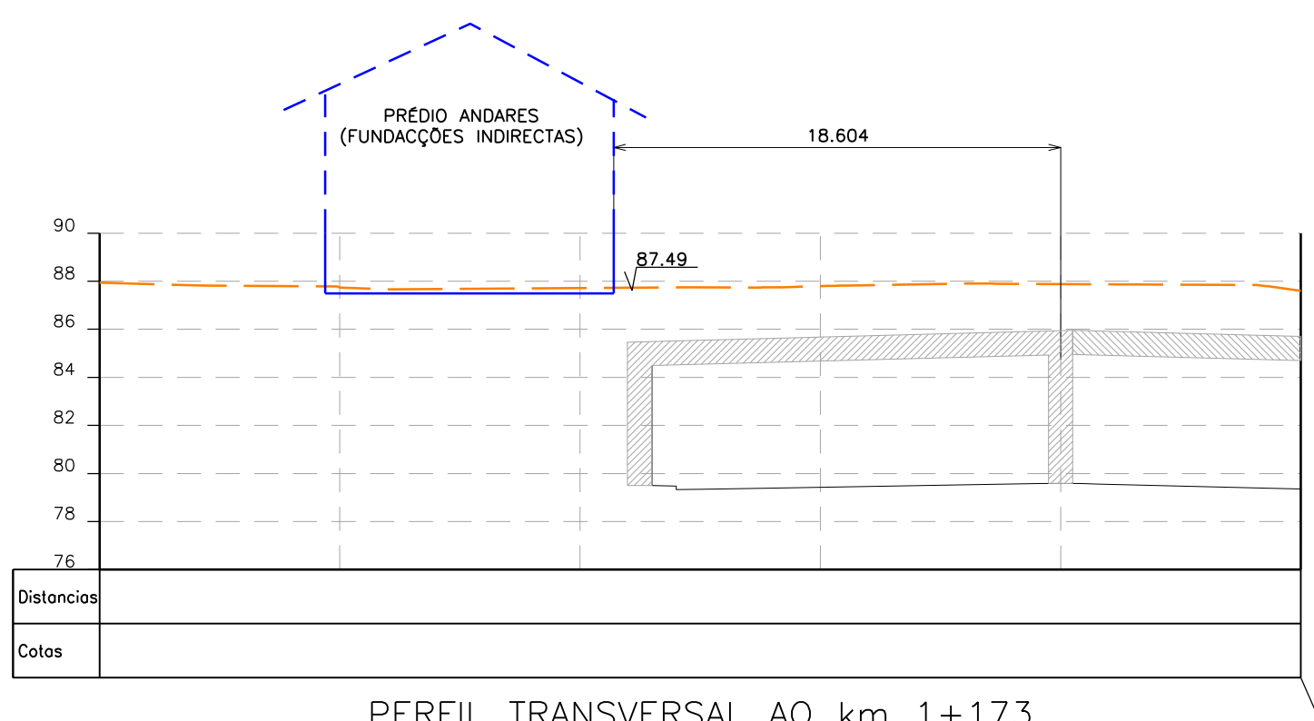
PERFIL TRANSVERSAL AO km 1+173
