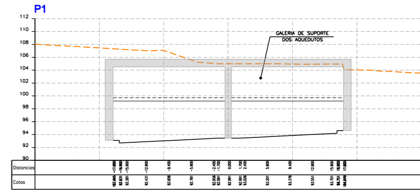
PERFIL TRANSVERSAL AO km 0+708,7
