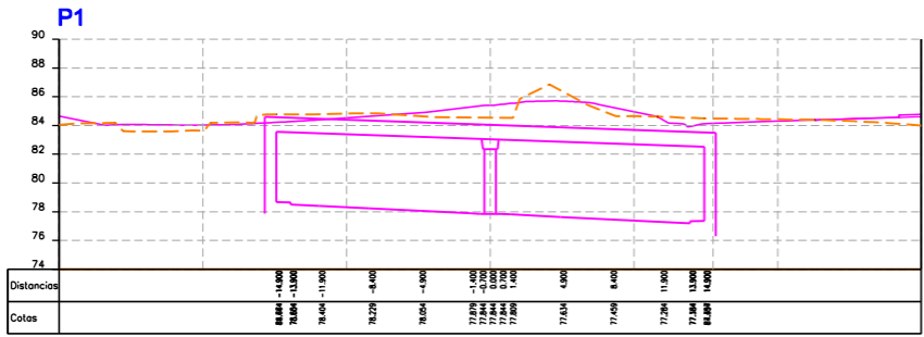
PERFIL TRANSVERSAL AO km 1+650
