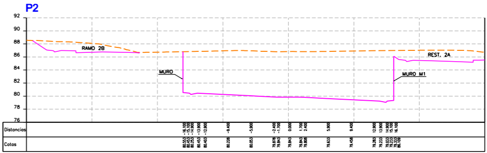
PERFIL TRANSVERSAL AO km 1+700
