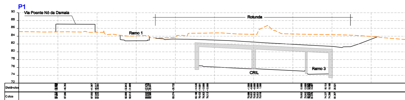
PERFIL TRANSVERSAL AO km 1+650
