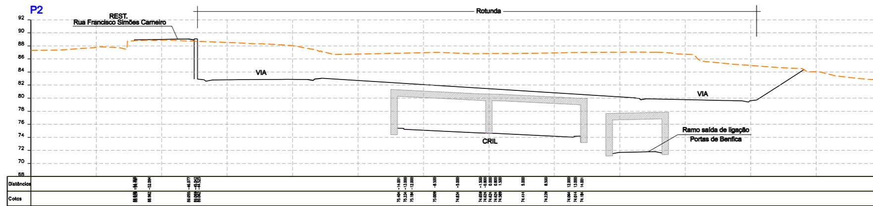
PERFIL TRANSVERSAL AO km 1+700
