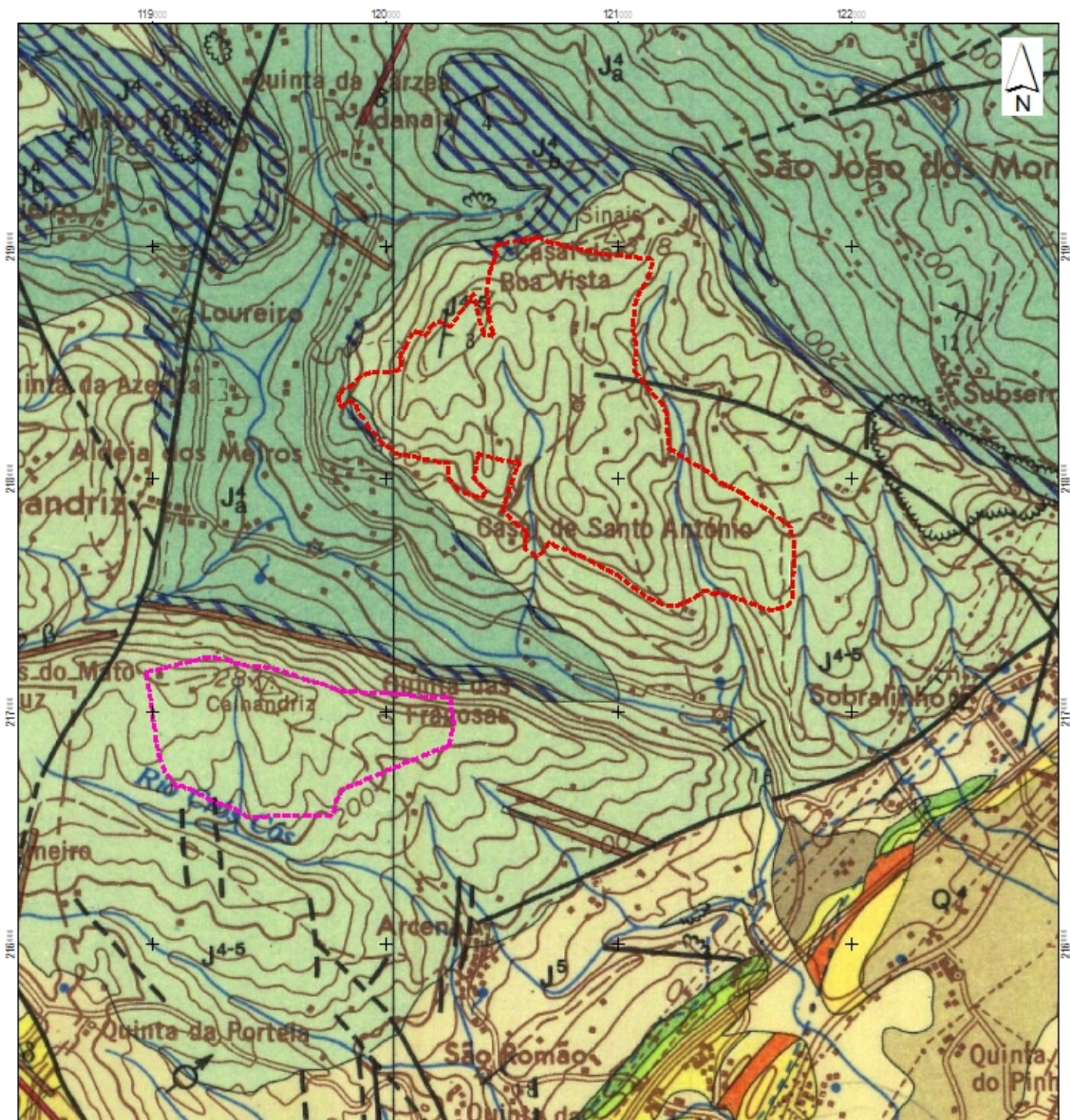
Fonte: Extracto da Carta Geológica de Portugal à Esc.:1:50 000, folha 34-B (Loures). Ampliada para a Esc.: 1:25 000. Coordenadas: Gauss-Elipsóide Internacional - Datum de Lisboa
