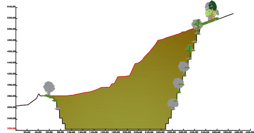
PERFIL 2
