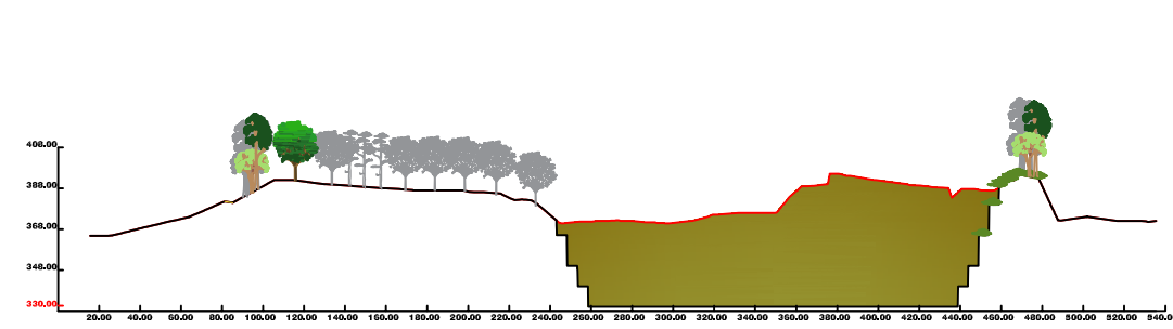
PERFIL 6
