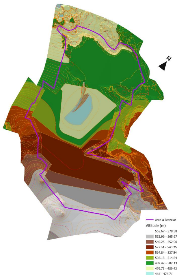
Figura 3-6 - Configuração da zona de extração (admitindo as profundidades máximas projetadas; note-se que a escombreira assinalada é provisória).
