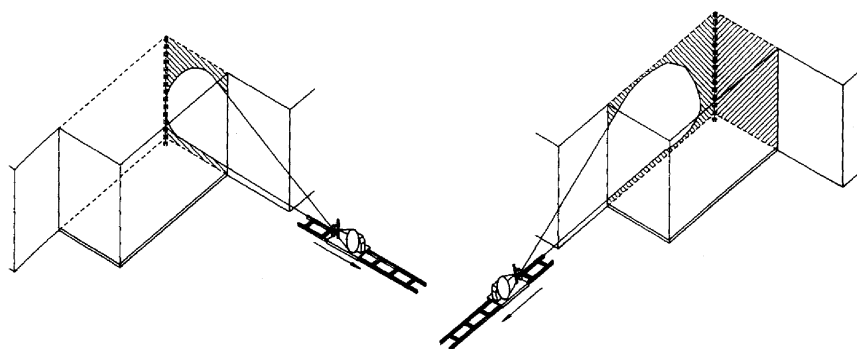
Figura 3-7 - Técnica de corte com fio diamantado.
