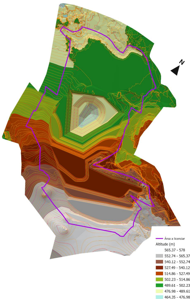
Figura 3-9 - Modelado topográfico após a modelação da zona explorada.
