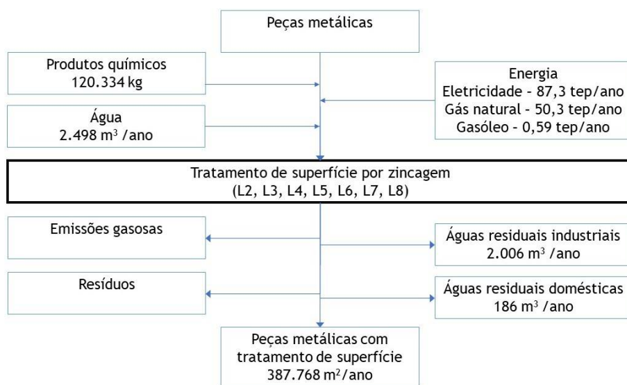
Figura 2 -- Representação esquemática do processo decorrente da ampliação proposta.
