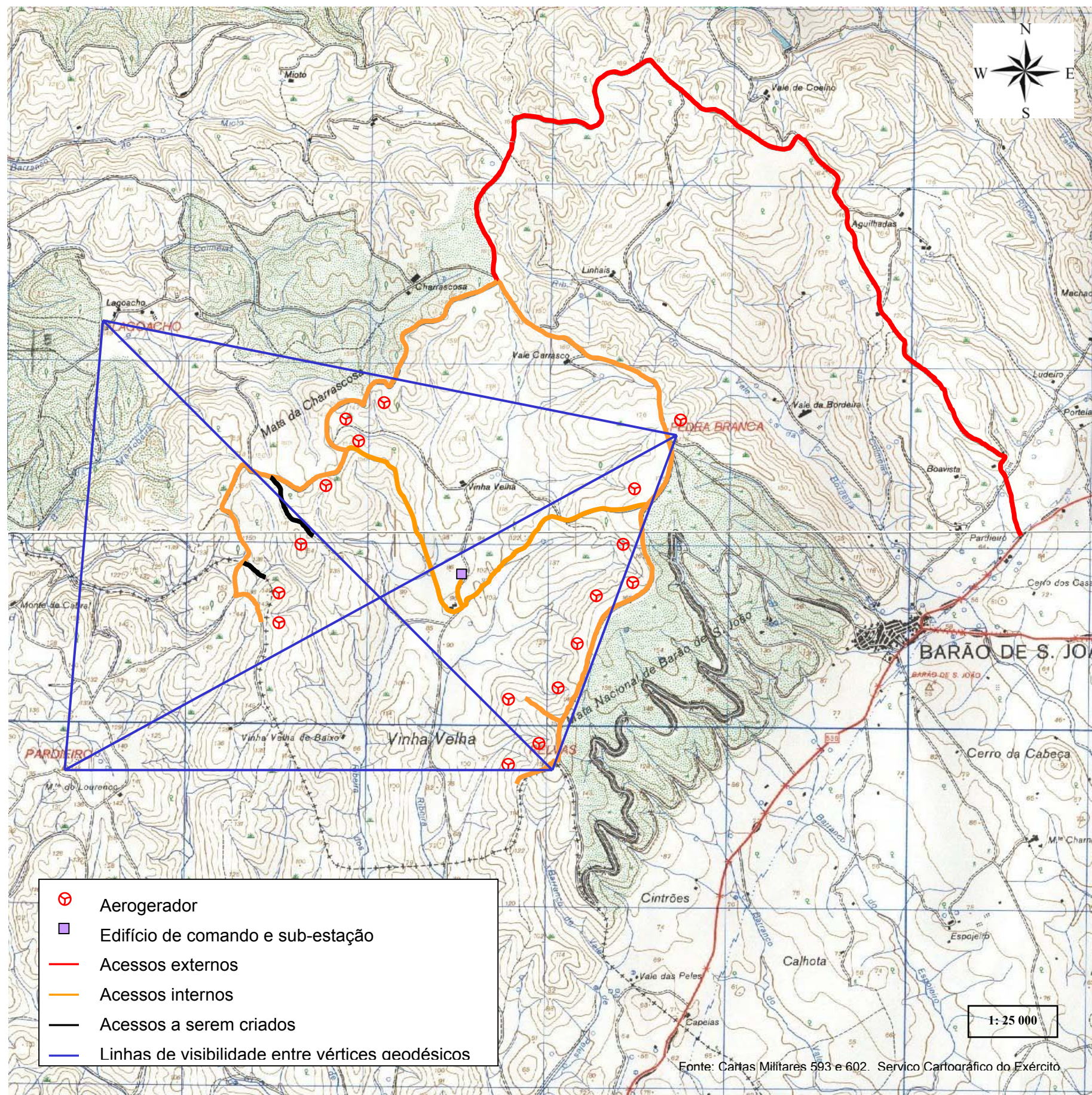
Figura 25 – Linhas de visibilidade entre vértices geodésicos
