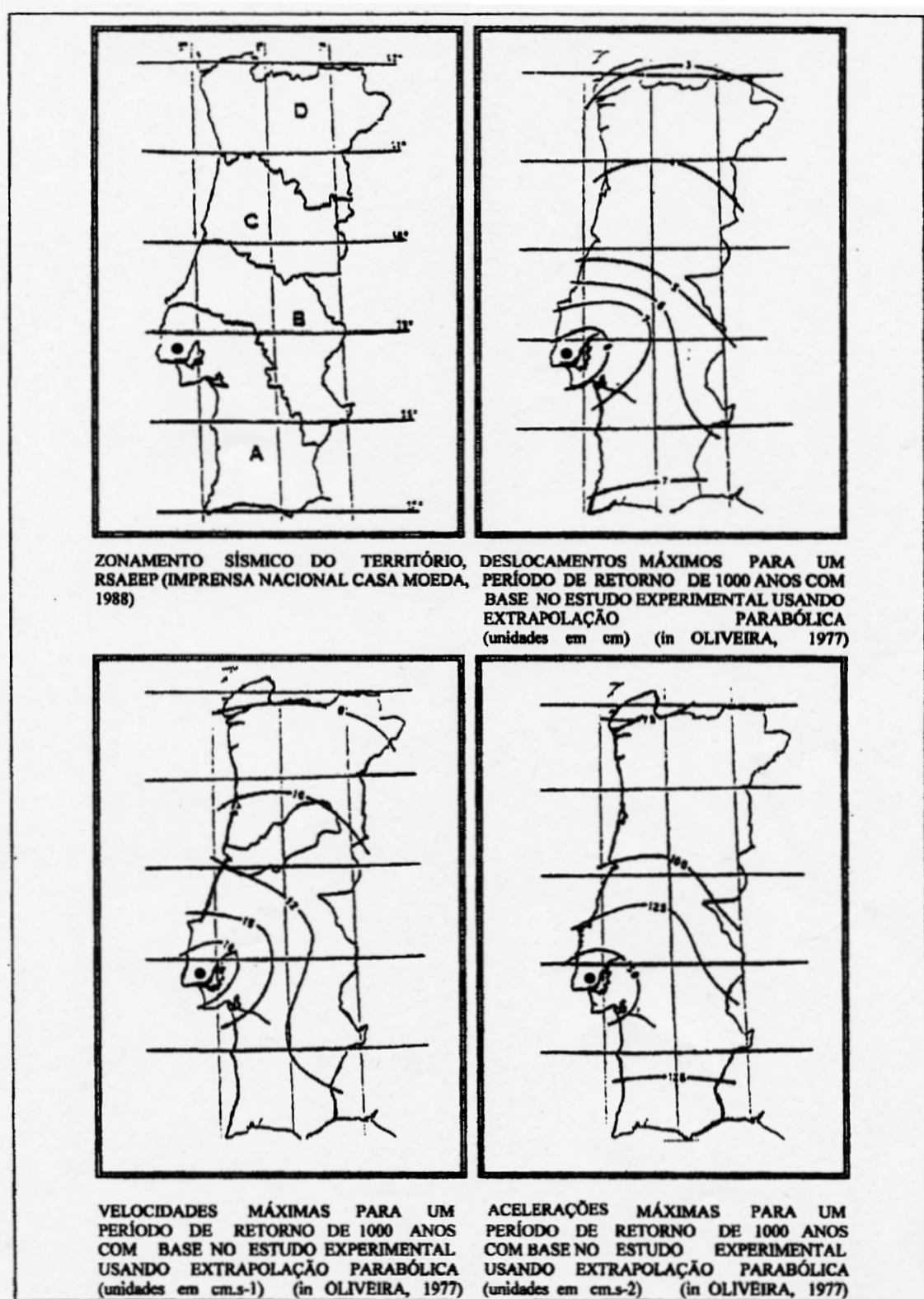
Figura 3 - Carta de Zonamentos de Riscos Sísmicos e Valores Máximos de Deslocamento, Velocidade e Aceleração
