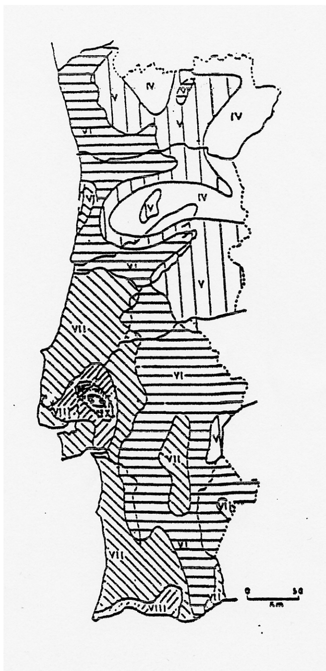
Figura 2 - Carta de Intensidades Sísmicas Fonte: Oliveira (1977)
