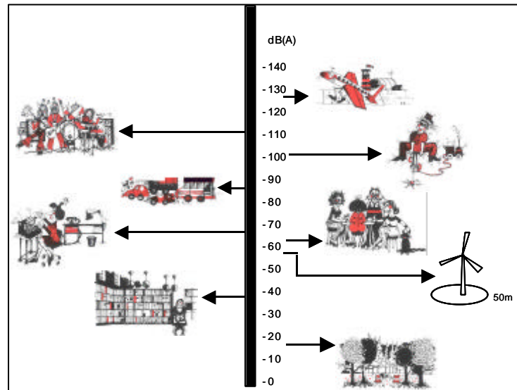
Figura 5 - Nível sonoro produzido por um aerogerador - comparação com níveis verificados para diferentes situações
