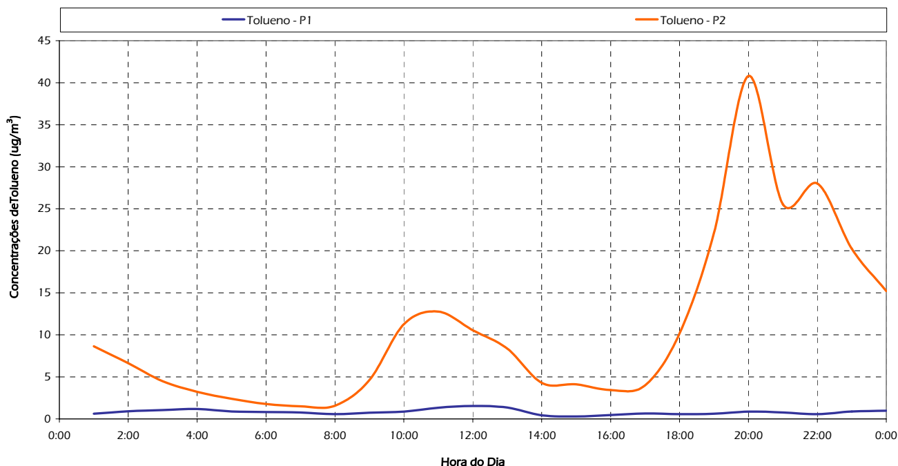
Figura 16 – Evolução média da variação horária das concentrações de Tolueno verificadas nas medições realizadas nos três pontos de medição.
