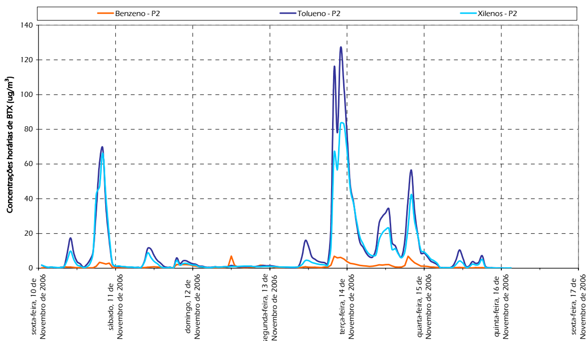
Figura 33 – Gráfico representativo dos resultados horários de Benzeno, Tolueno e Xilenos (NA) obtidos no Ponto P2.
