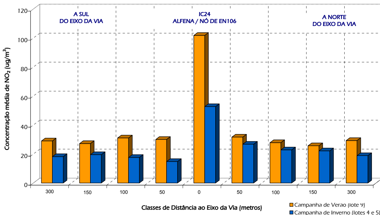
Figura 6 – Valores médios de NO 2 por distância ao eixo da via no IC24 Alfena/ Nó de EN 106.
