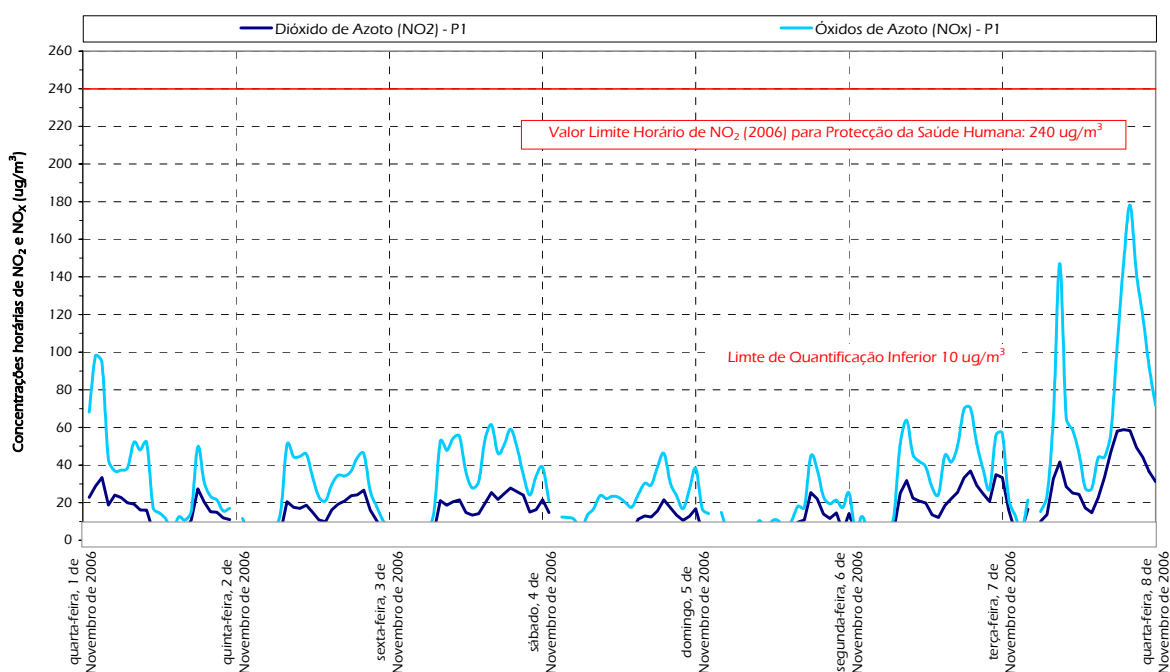
Figura 20 – Gráfico representativo dos resultados horários de Dióxido de Azoto (A) e Óxidos de Azoto (A) obtidos no Ponto P1.
