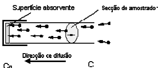
Figura 5 – Vista esquemática de um amostrador passivo.
