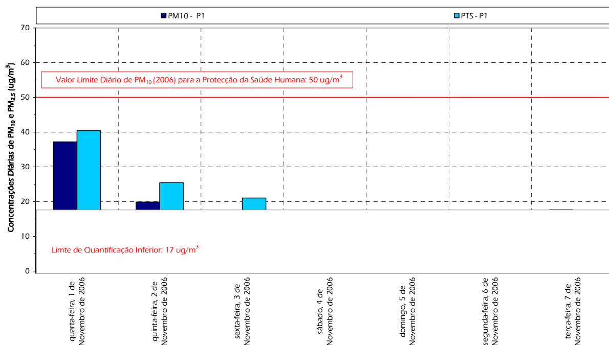
Figura 30 – Gráfico representativo dos resultados diários de PM 10 e PTS (A) obtidos no Ponto P1.
