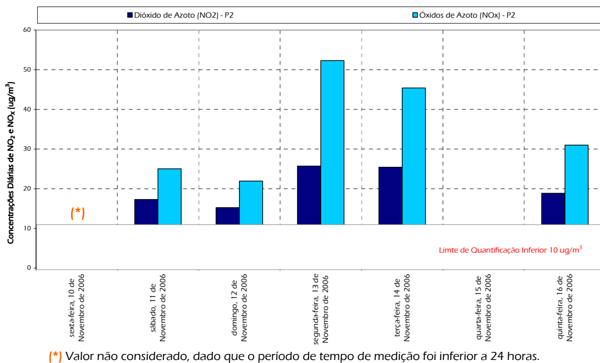
Figura 23 – Gráfico representativo dos resultados diários de Dióxido de Azoto (A) e Óxidos de Azoto (A) obtidos no Ponto P2.
