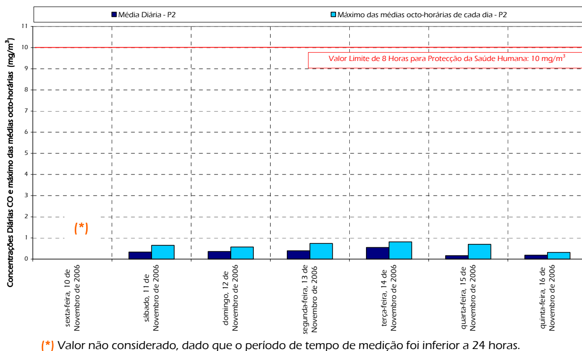
Figura 27 – Gráfico representativo dos resultados máximos octo-horários e diários de Monóxido de Carbono (A) obtidos no Ponto P2.
