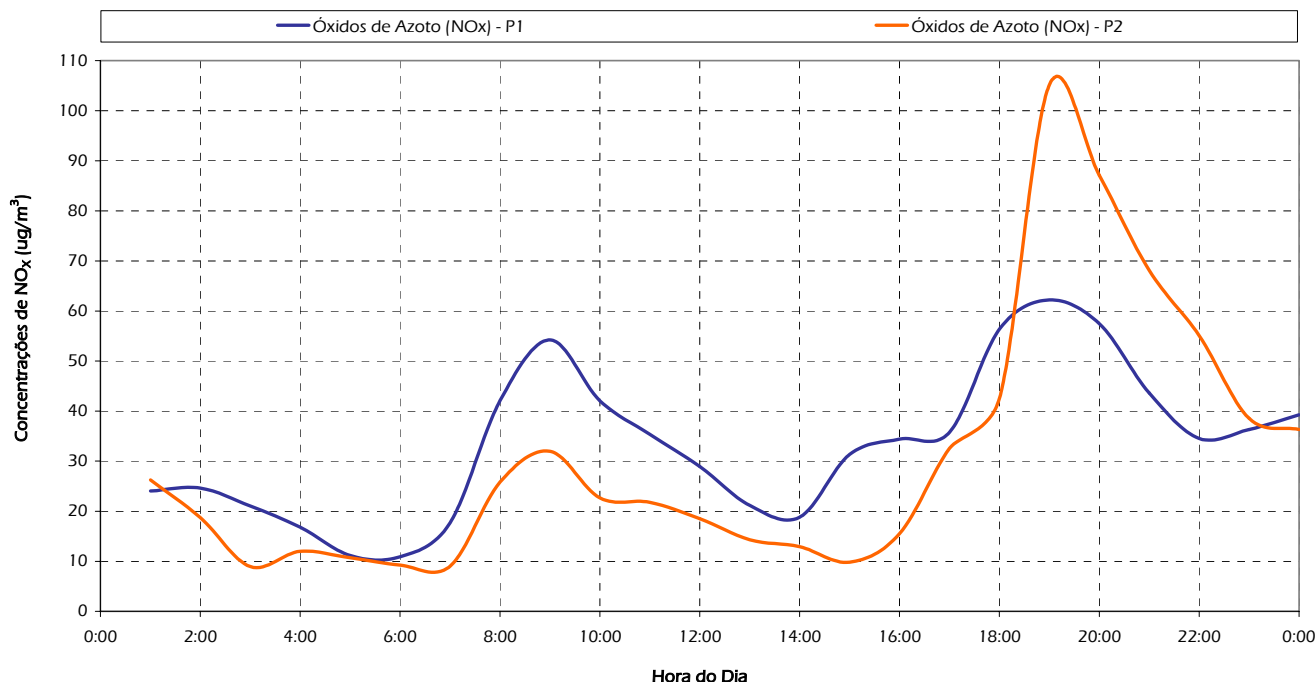
Figura 11 – Evolução média da variação horária das concentrações de NO x verificadas nas medições realizadas nos dois pontos de medição.
