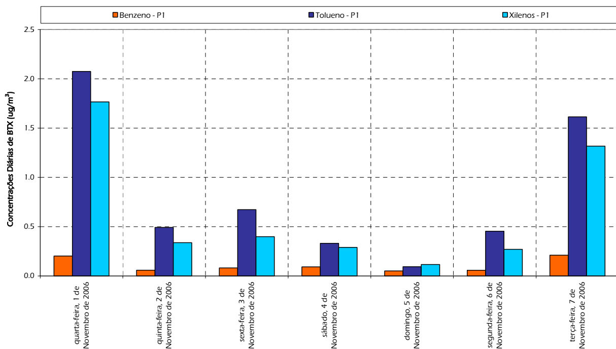
Figura 34 – Gráfico representativo dos resultados diários de Benzeno, Tolueno e Xilenos (NA) obtidos no Ponto P1.
