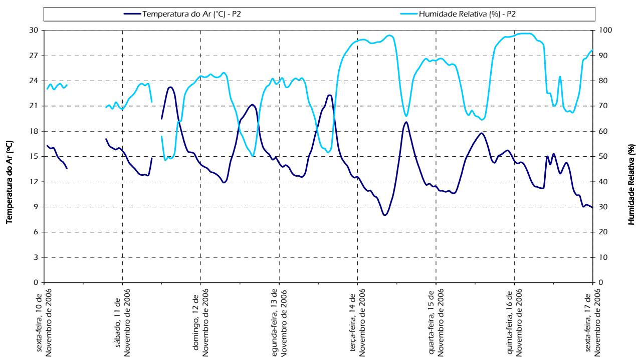
Figura 39 – Variação temporal das médias horárias de temperatura do ar e humidade relativa durante as medições ocorridas no Ponto P2.
