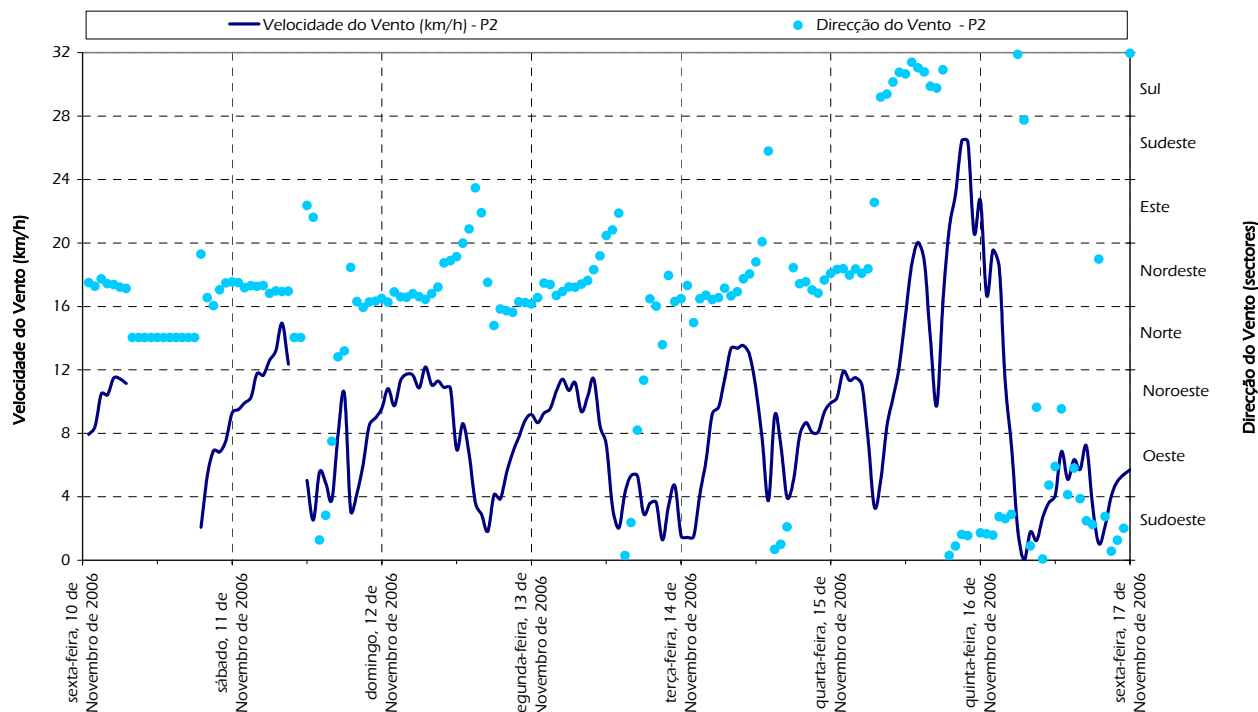
Figura 41 – Variação temporal das médias horárias de direcção e velocidade do vento durante as medições ocorridas no Ponto P2.
