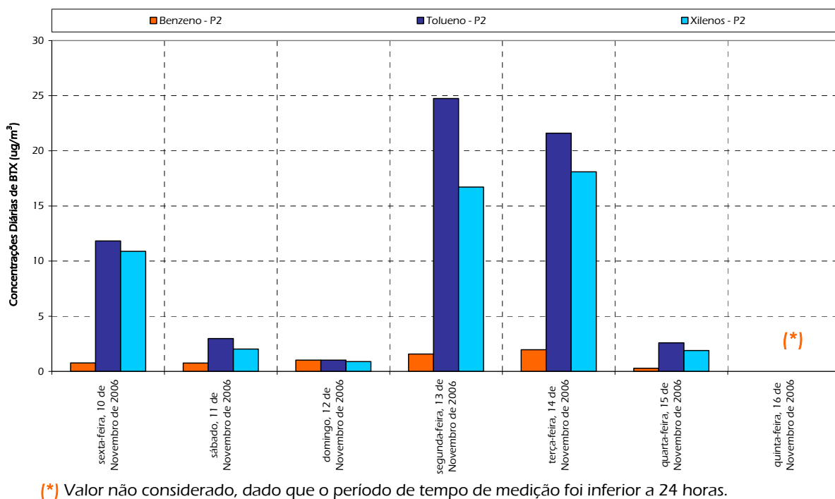
Figura 35 – Gráfico representativo dos resultados diários de Benzeno, Tolueno e Xilenos (NA) obtidos no Ponto P2.
