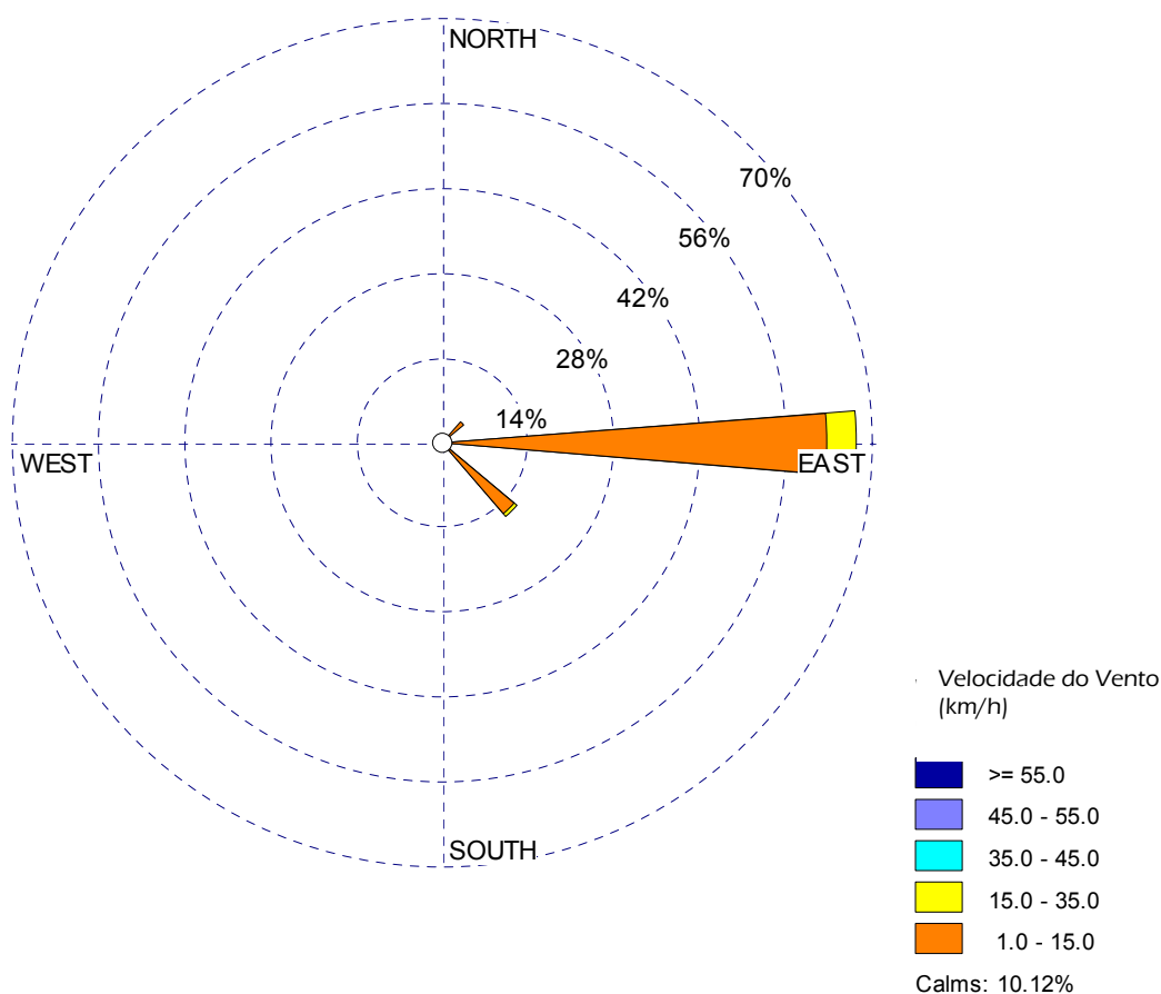
Figura 42 – Rosa de ventos relativa às observações horárias de velocidade e direcção do vento ocorridas no Ponto P1.
