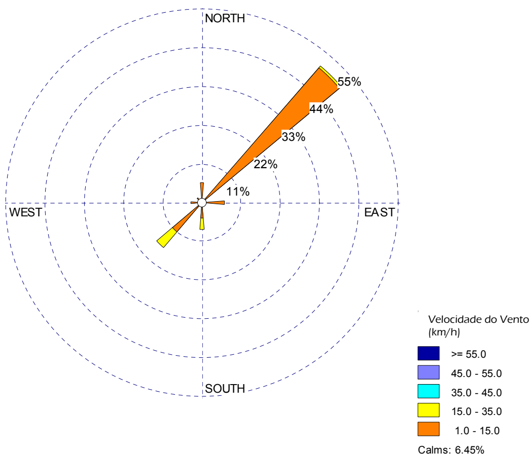
Figura 43 – Rosa de ventos relativa às observações horárias de velocidade e direcção do vento ocorridas no Ponto P2.
