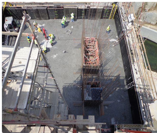
Foto 2.3.10 – Ribeiradio – Barragem – Betonagem do Bloco 10.
