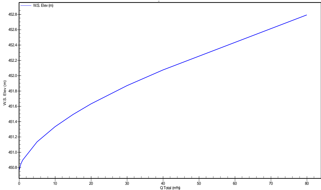
Figura 1 – Curva de Vazão, para T=100 anos.
