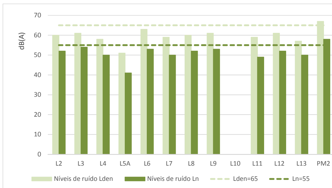
Figura 4 – Comparação dos indicadores L_{den} e L_n obtidos no sublaço Carcavelos / Estoril com os respetivos limites legais aplicáveis
