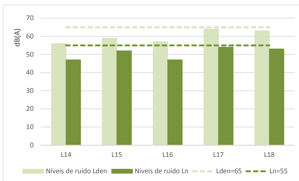
Figura 5 – Comparação dos indicadores L_{den} e L_n obtidos no sublaço Estoril / Alcabideche com os respetivos limites legais aplicáveis
