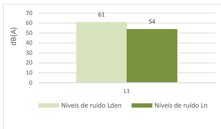
Figura 3 – Comparação dos indicadores L_{den} e L_n obtidos no sublaço Oeiras / Carcavelos com os respetivos limites legais aplicáveis
