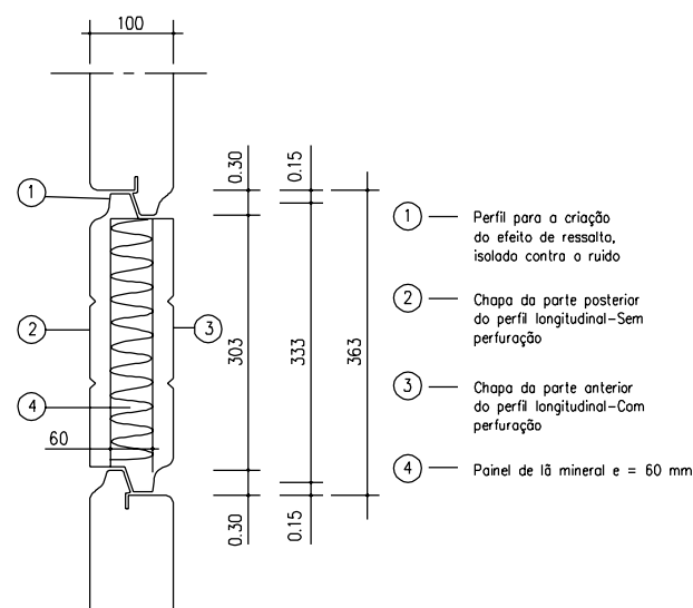
PORMENOR DO PAINEL METÁLICO
