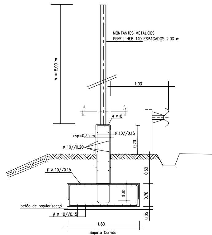
PERFIL TRANSVERSAL TIPO DA BARREIRA
