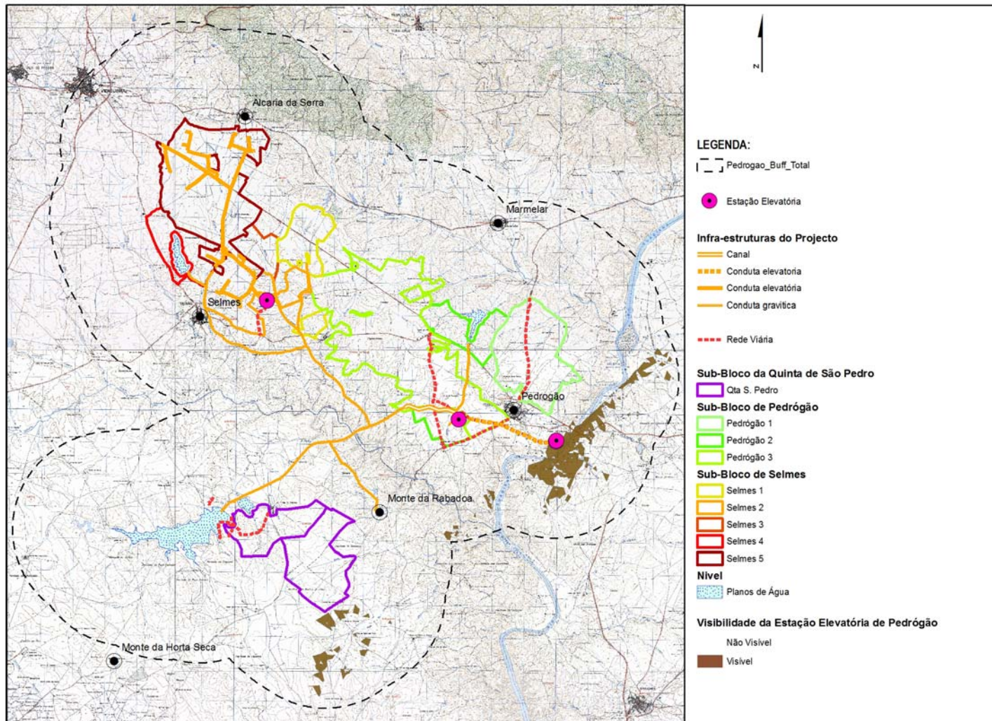
Figura 2.3 – Bacia visual da estação elevatória principal de Pedrógão.
