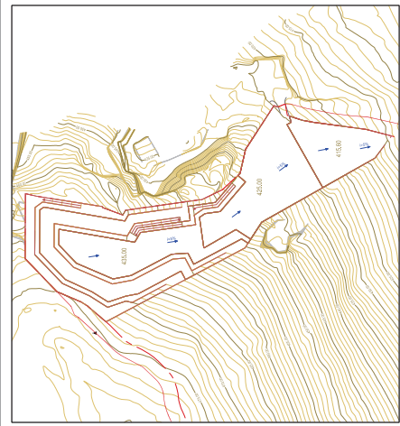
PLANTA ESQUEMÁTICA DE DRENAGEM DO PATAMAR BASE DA ZONA A (ÁREA DE EXPLORAÇÃO A CÉU ABERTO).
