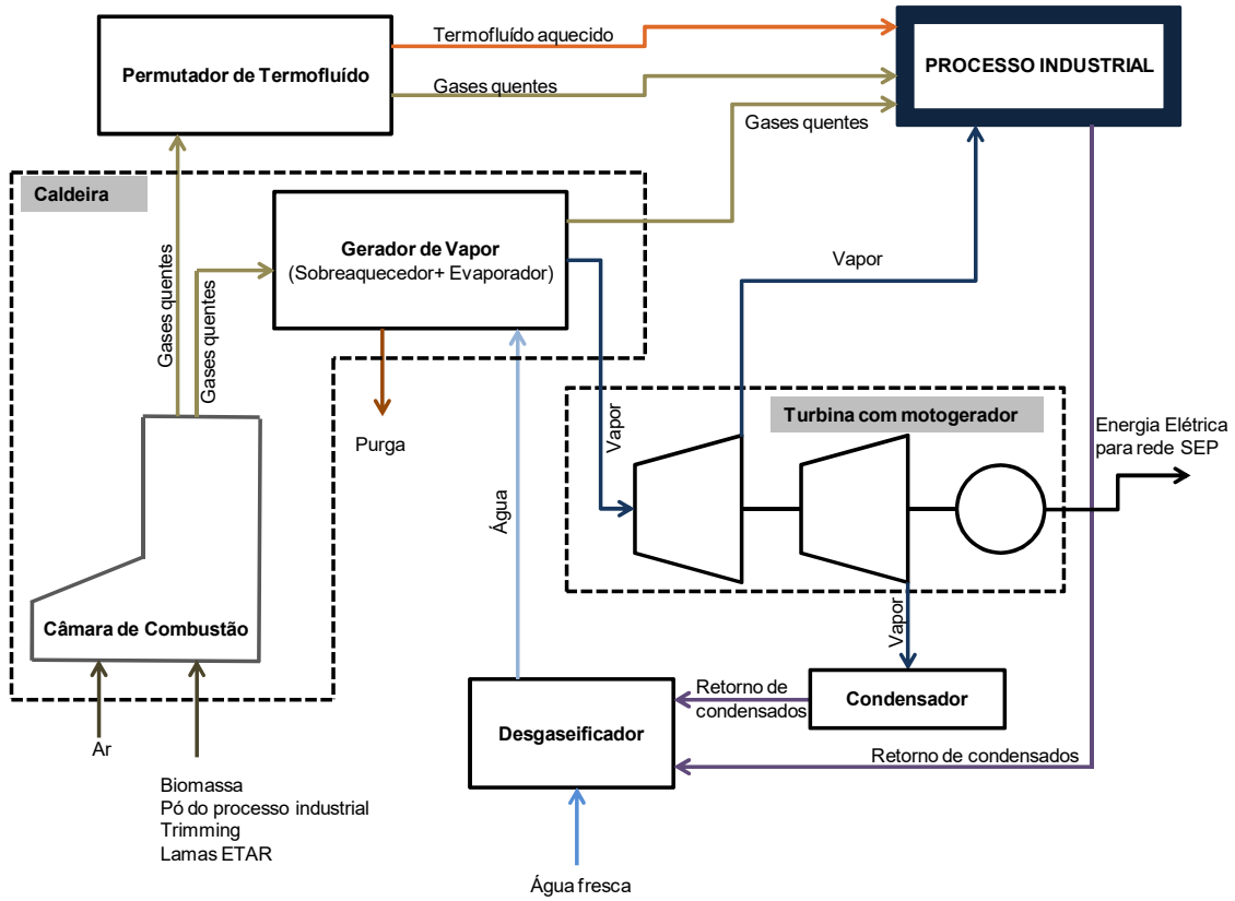
Ilustração 1 - Fluxograma produtivo da actividade desenvolvida
