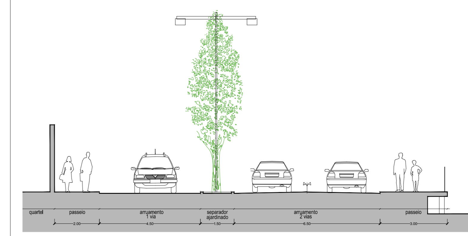
PERFIL A - A' Esc. 1/100
