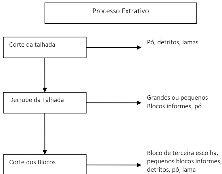
Figura 110. Esquema típico de produção de resíduos no processo extrativo.
