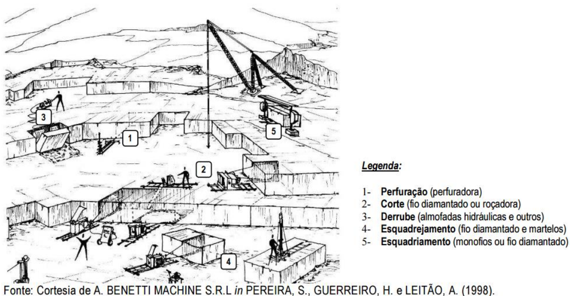
Figura 21. Operações realizadas numa pedreira de rocha ornamental a céu aberto.
