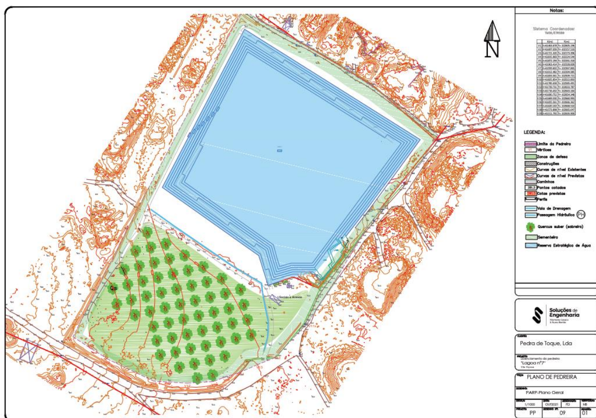
Figura 22. Plano Geral de Recuperação proposto para a Pedreira “Lagoa nº7” (Fonte: PARP).
