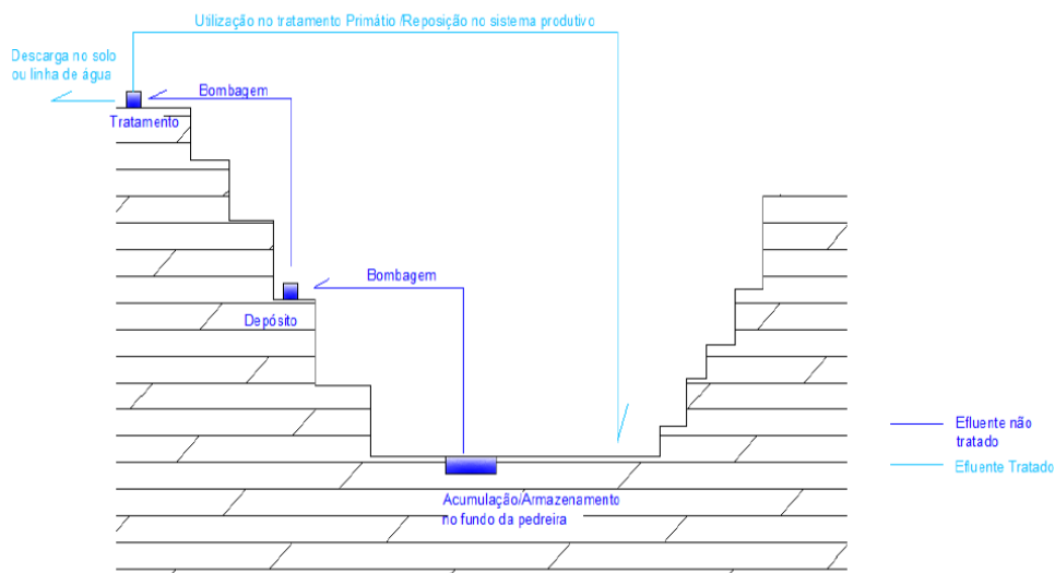
Figura 56. Representação esquemática de um sistema de recirculação de água numa pedreira, de mármore, típica.
