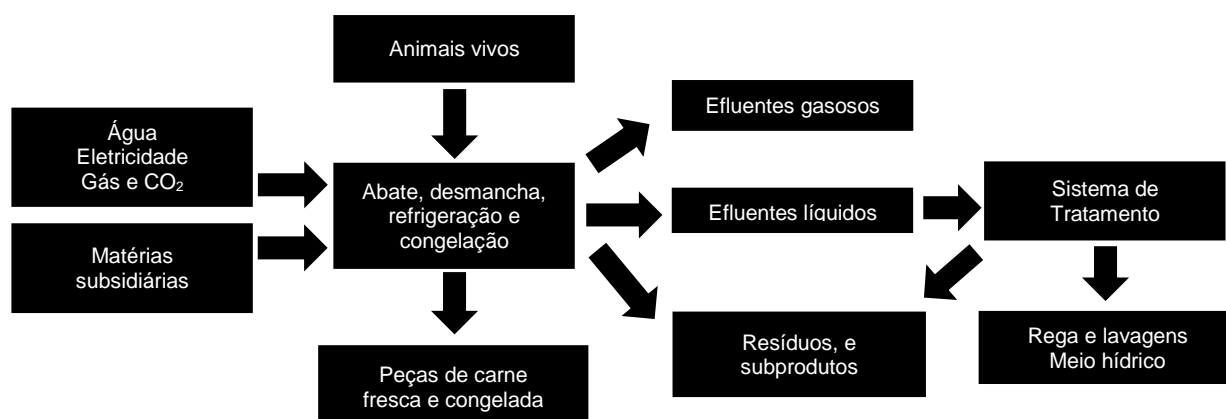
Figura 7 – Representação esquemática do processo produtivo.
