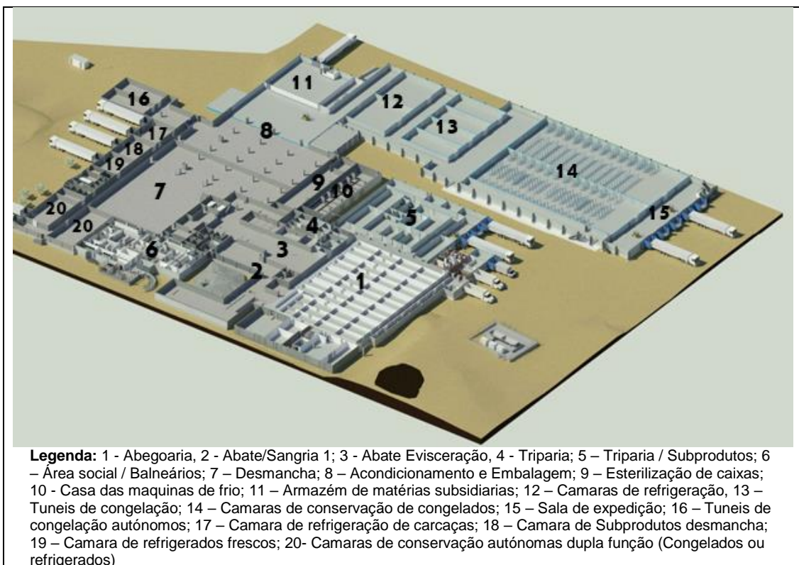
Figura 3 – Visualização da configuração final da Maporal – distribuição de atividades – piso 0
