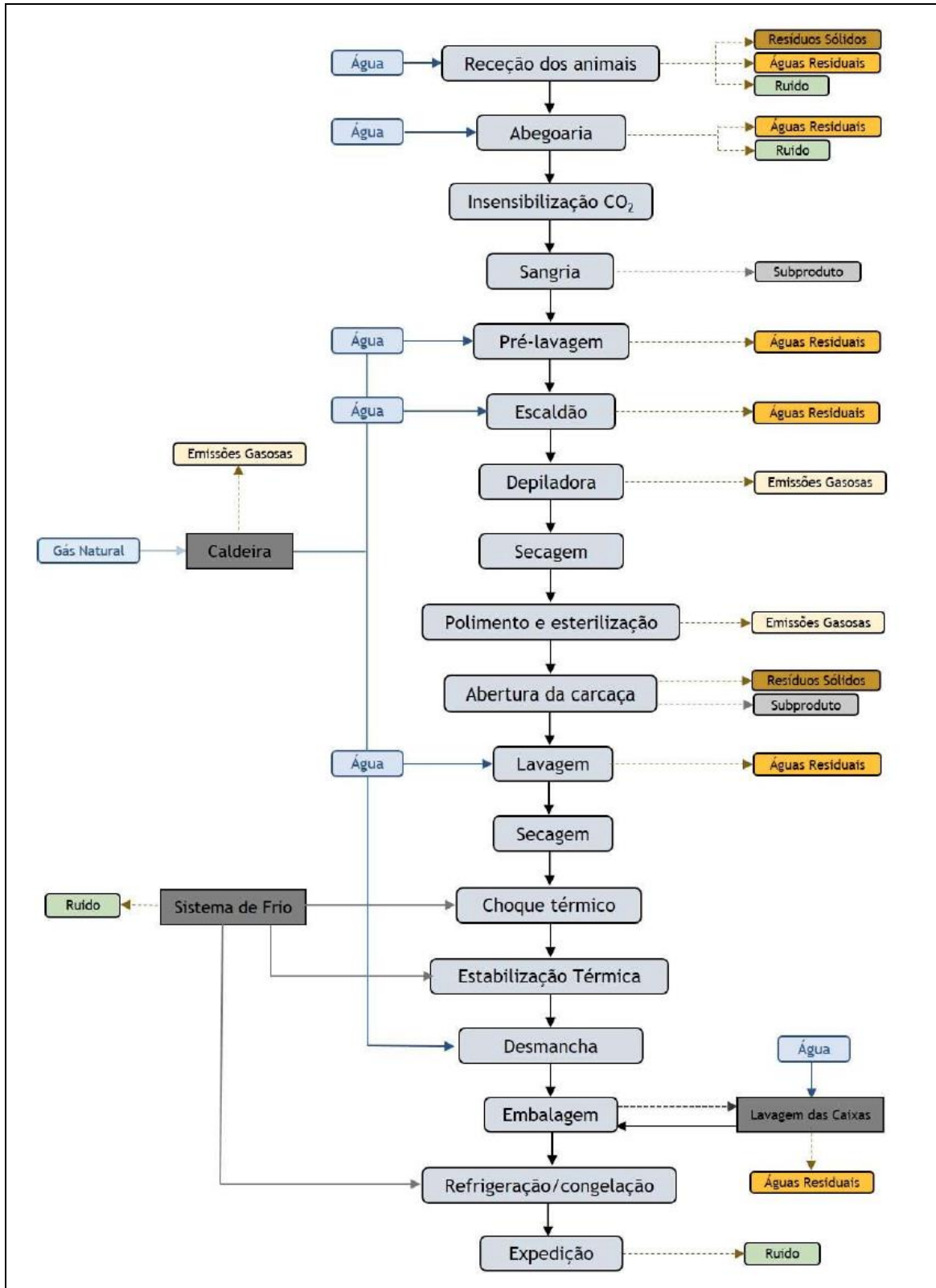
Figura 5 – Fluxograma do processo produtivo.
