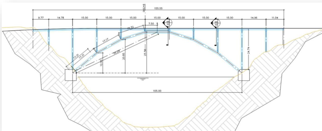
Imagen 1. Corte longitudinal del puente sobre el río Sever
