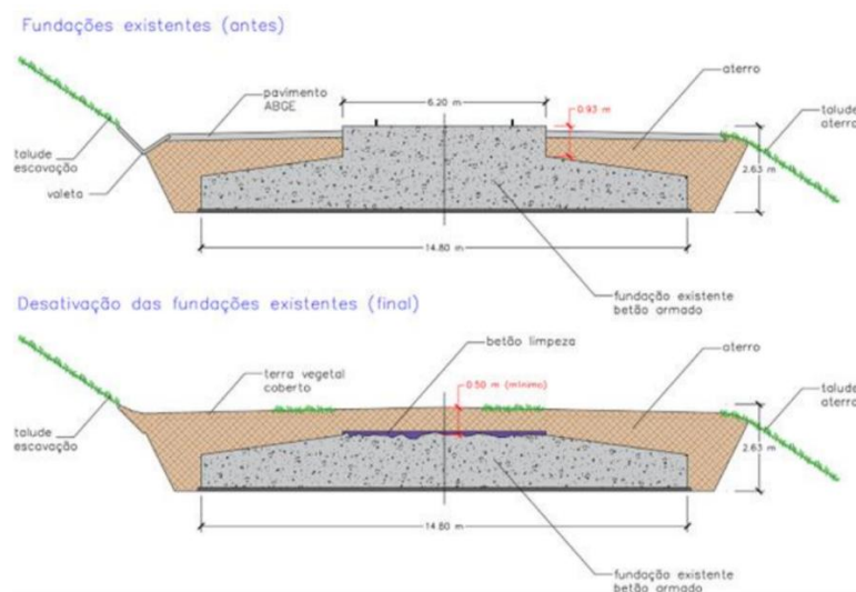
Figura 1 - Fundações existentes Vs. Fundações desativadas. Fonte: Resposta ao PEU
