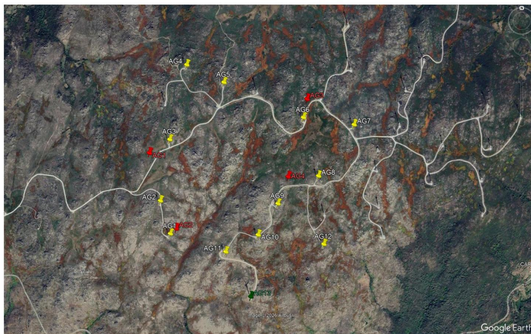
Figura 2 - Parque Eólico de Pinheiro - Marcação de todos os aerogeradores (a desmontar a amarelo, futuros a vermelho, a manter a verde) (Google Earth)
