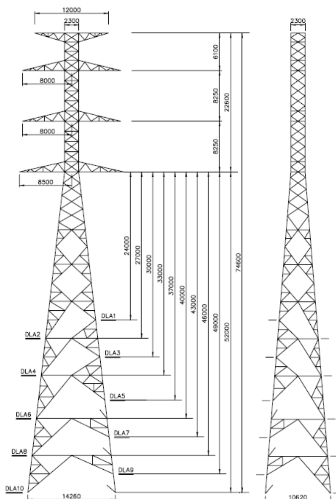
Figura 4.9 – Tipo de apoio da família “DL”
