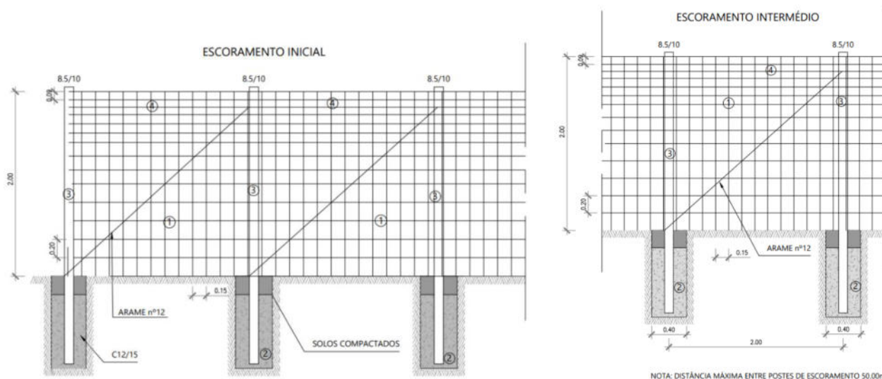
Figura 4.6 – Detalhes da vedação proposta
