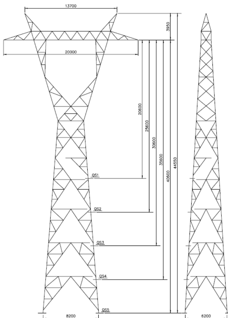
Figura 4.8 – Tipo de apoio da família "Q"
