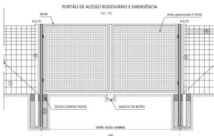
Figura 4.7 – Detalhes dos portões propostos
