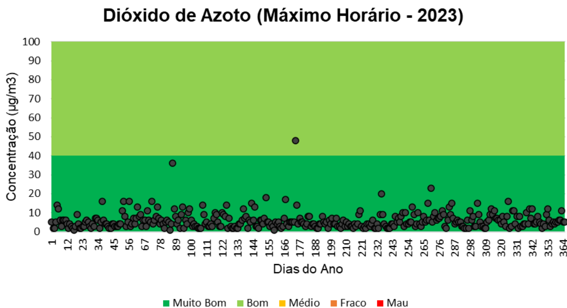
Figura 12.5 – Distribuição anual das emissões de \text{NO}_2 para a estação de Santiago do Cacém.
