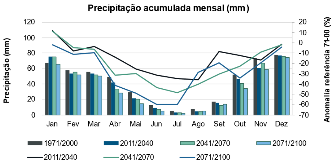
Figura 2.18 – Precipitação acumulada mensal simulada utilizando o RCP 8.5 para os intervalos de tempo 1971-2000, 2011-2040, 2041-2070 e 2071-2100 e sua respetiva anomalia.
