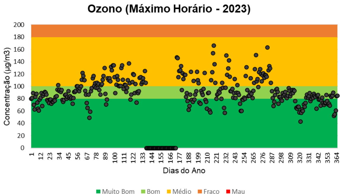
Figura 12.4 – Distribuição anual das emissões de \text{O}_3 para a estação de Santiago do Cacém.
