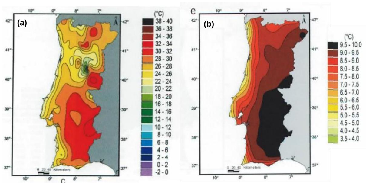
Figura 2.10 – Temperatura máxima de verão (Portugal Continental) sendo em (a) simulação de controlo (1961-1990) e em (b) projeção de acordo com cenário de emissões A2 (2071-2100).
