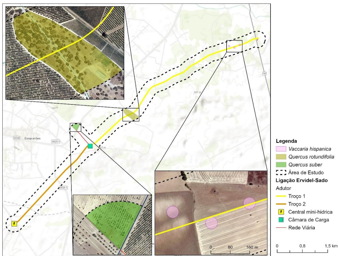
Figura 7.6 – Locais onde foi detetada a presença da espécie ameaçada flor-das-vacas ( Vaccaria hispanica var. hispânica ) e das espécies protegidas azinheira ( Quercus rotundifolia ) e sobreiro ( Quercus suber ).
