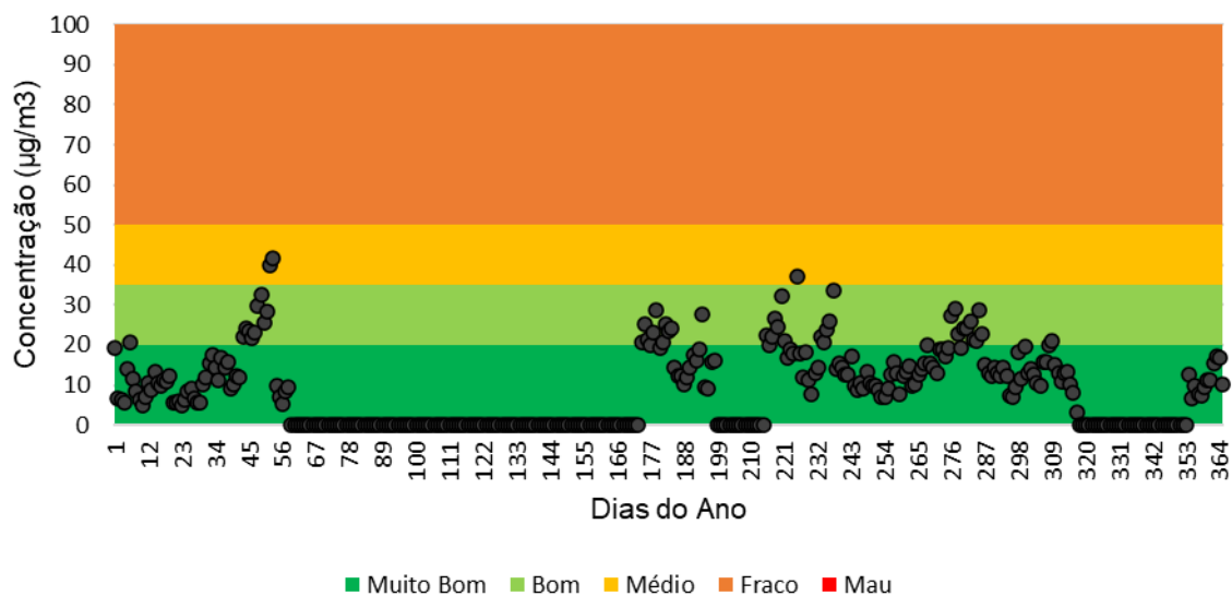
Figura 12.7 – Distribuição anual das emissões de PM 10 para a estação de Santiago do Cacém.
