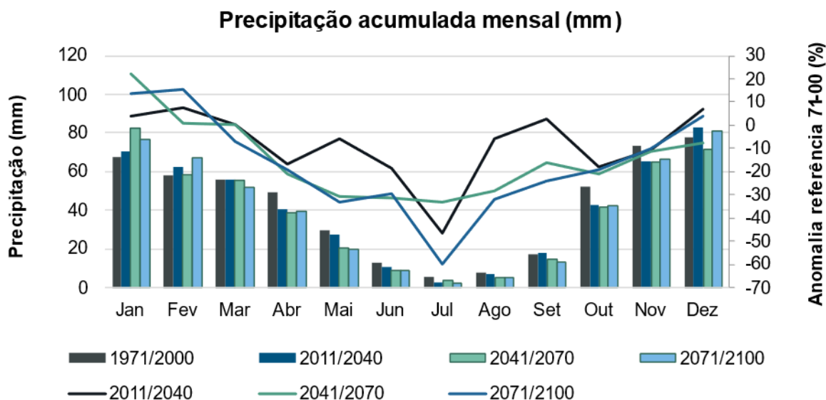
Figura 2.17 – Precipitação acumulada mensal simulada utilizando o RCP 4.5 para os intervalos de tempo 1971-2000, 2011-2040, 2041-2070 e 2071-2100 e sua respetiva anomalia.
