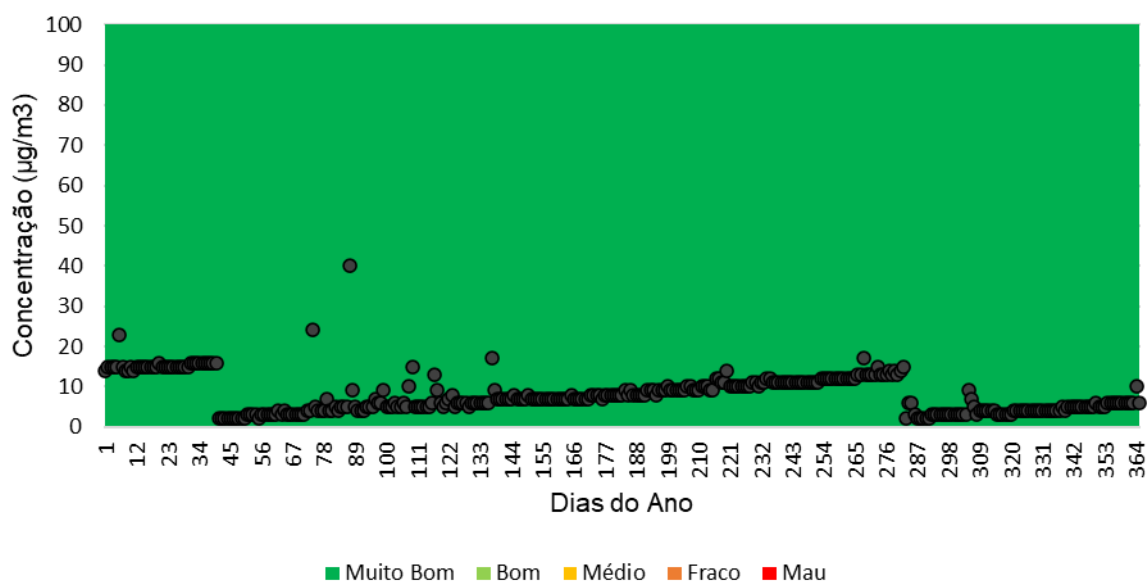
Figura 12.6 – Distribuição anual das emissões de SO 2 para a estação de Santiago do Cacém.
