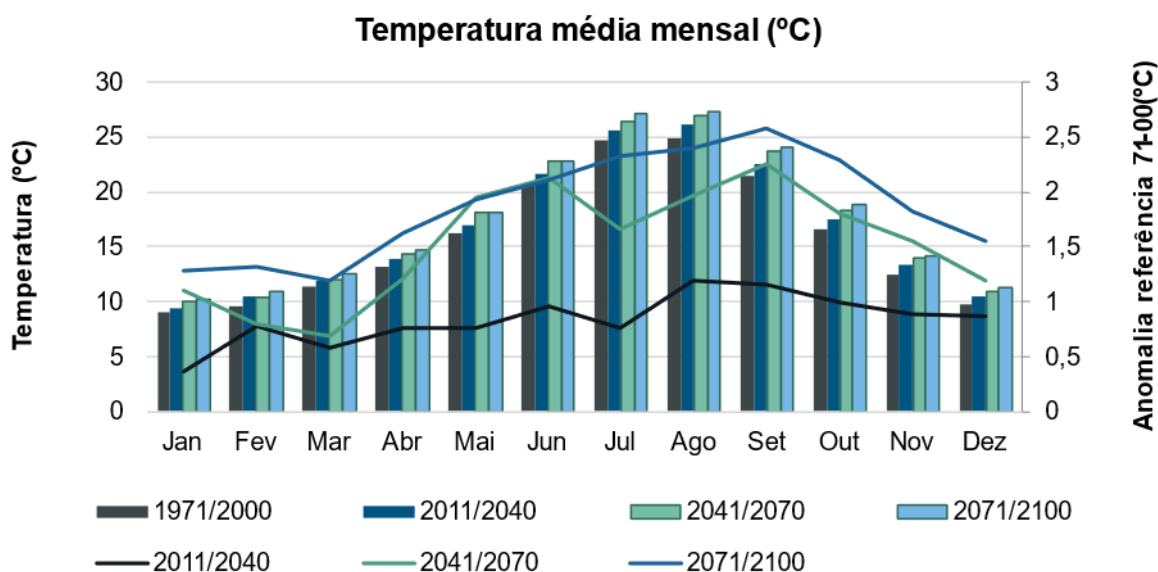
Figura 2.12 – Temperatura média mensal simulada utilizando o RCP 4.5 para os intervalos de tempo 1971-2000, 2011-2040, 2041-2070 e 2071-2100, e sua respetiva anomalia.
