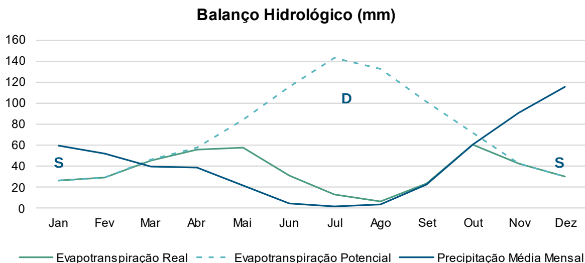
Figura 2.9 – Balanço hidrológico, onde a letra “S” indica as zonas de superávit hídrico e a letra “D” indica as zonas de defícite hídrico.
