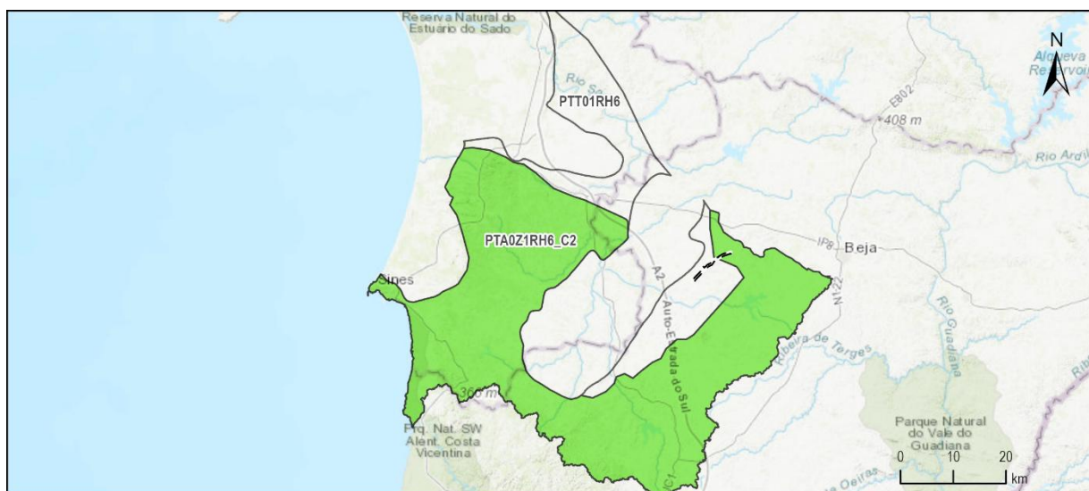
Figura 4.9 – Carga anual de CBO 5 por massa de água subterrânea existente na área de estudo de origem na indústria extrativa.
