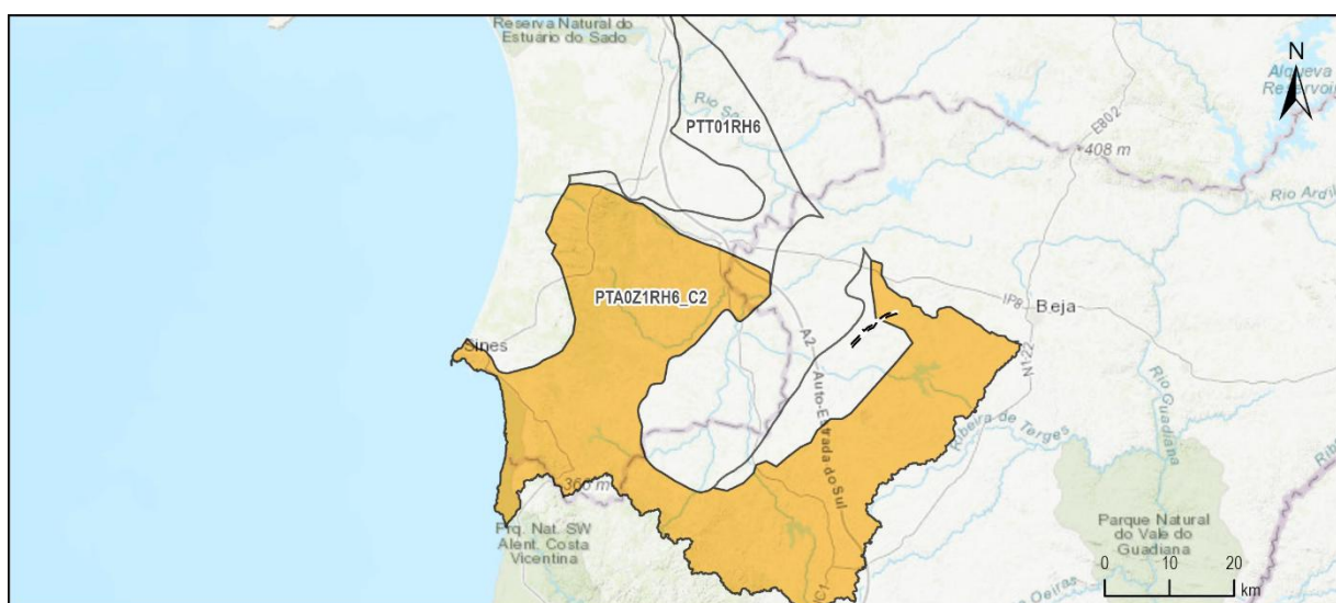
Figura 4.14 – Carga anual de CQO por massa de água subterrânea existente na área de estudo de origem no setor do turismo.
