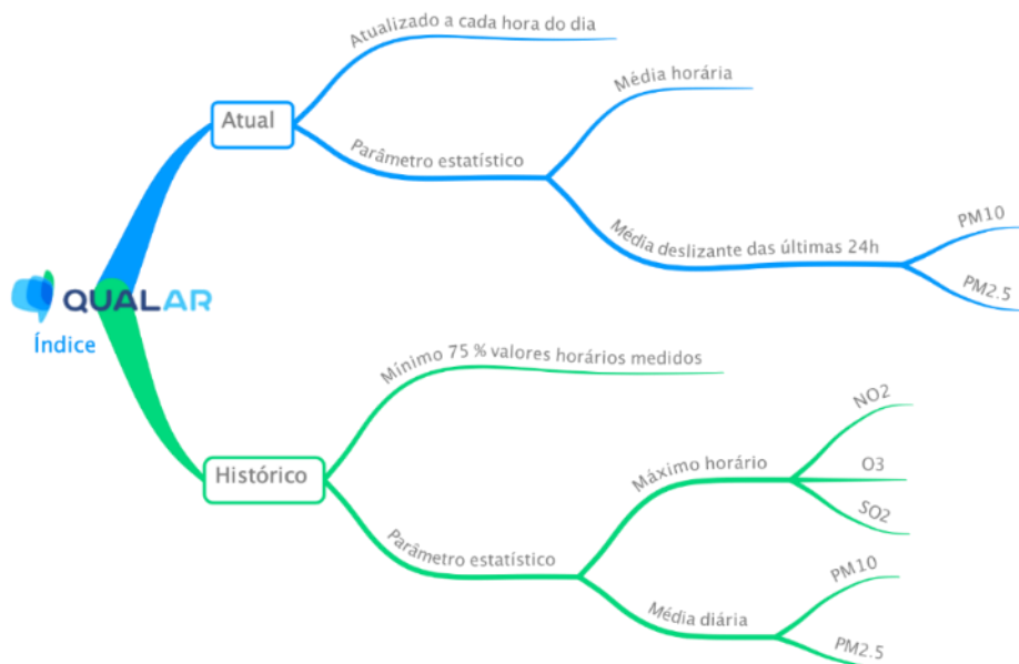
Figura 12.3 – Método de cálculo do IQar. (Fonte: Qualar – Informação sobre qualidade do ar)
