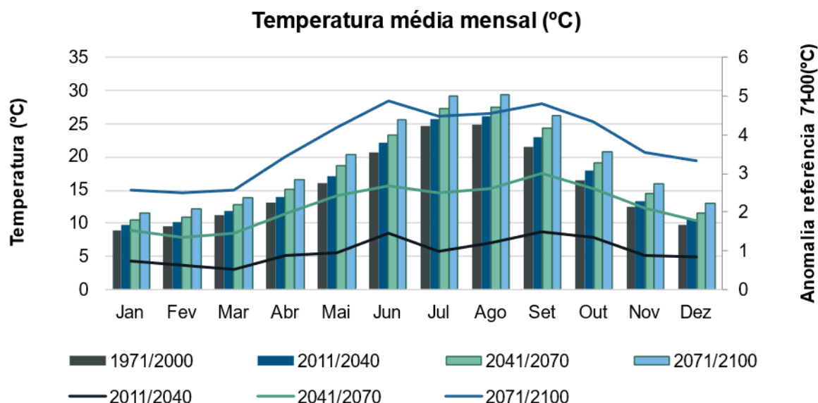
Figura 2.13 – Temperatura média mensal simulada utilizando o RCP 8.5 para os intervalos de tempo 1971-2000, 2011-2040, 2041-2070 e 2071-2100 e sua respetiva anomalia.
