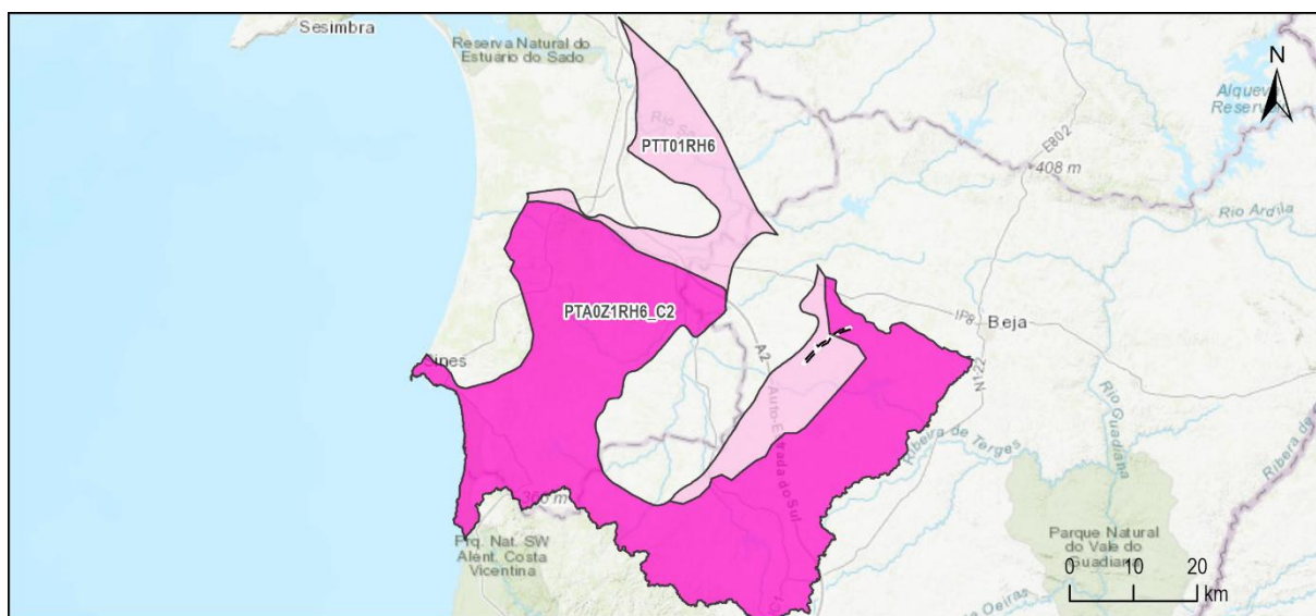
Figura 4.19 – Carga anual de azoto por massa de água subterrânea existente na área de estudo de origem agrícola.
