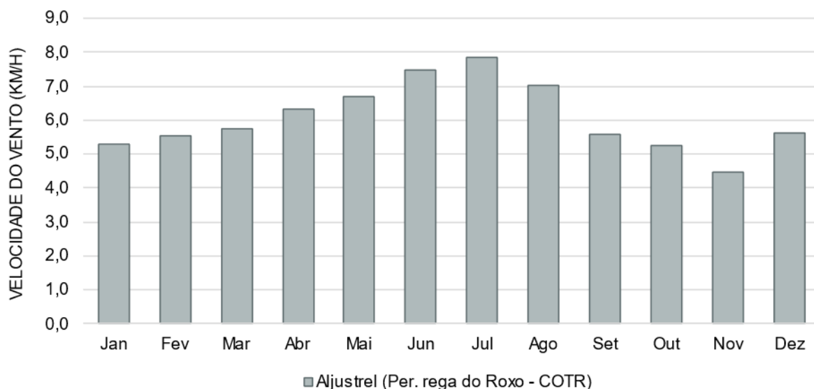
Figura 2.6 – Velocidade média do vento.
