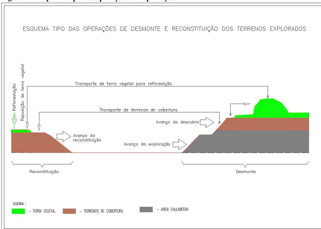
Figura 1 – Esquema tipo das operações de exploração.
