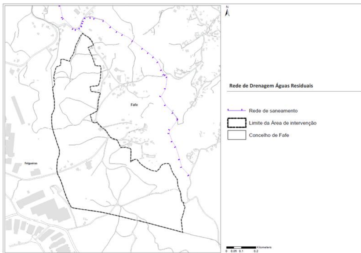
Figura 18 – Rede de drenagem de águas residuais.
