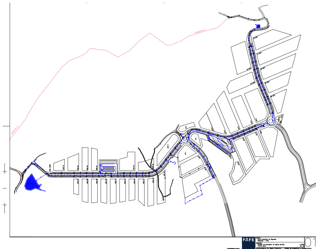
Figura 19 – Projeto da Rede de Águas Pluviais.
