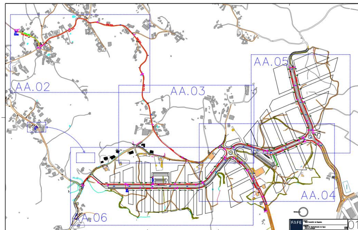
Figura 17 – Projeto da Rede de Abastecimento de Água.
