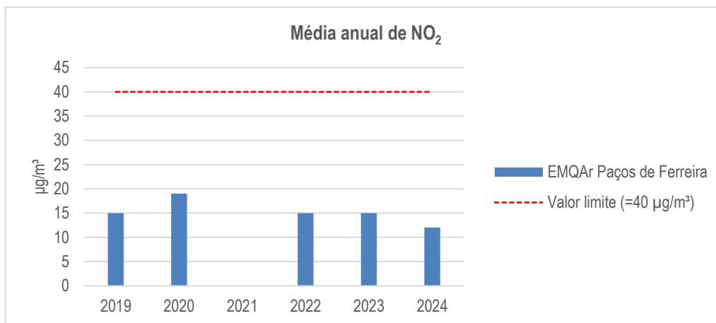
Figura 122 – Dados estatísticos da EMQAr de Paços de Ferreira relativos às concentrações médias anuais de NO 2 entre 2019 e 2024.
