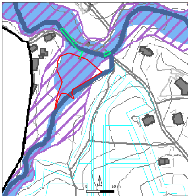
(a) Bacia de Retenção norte (BR2) e PH
