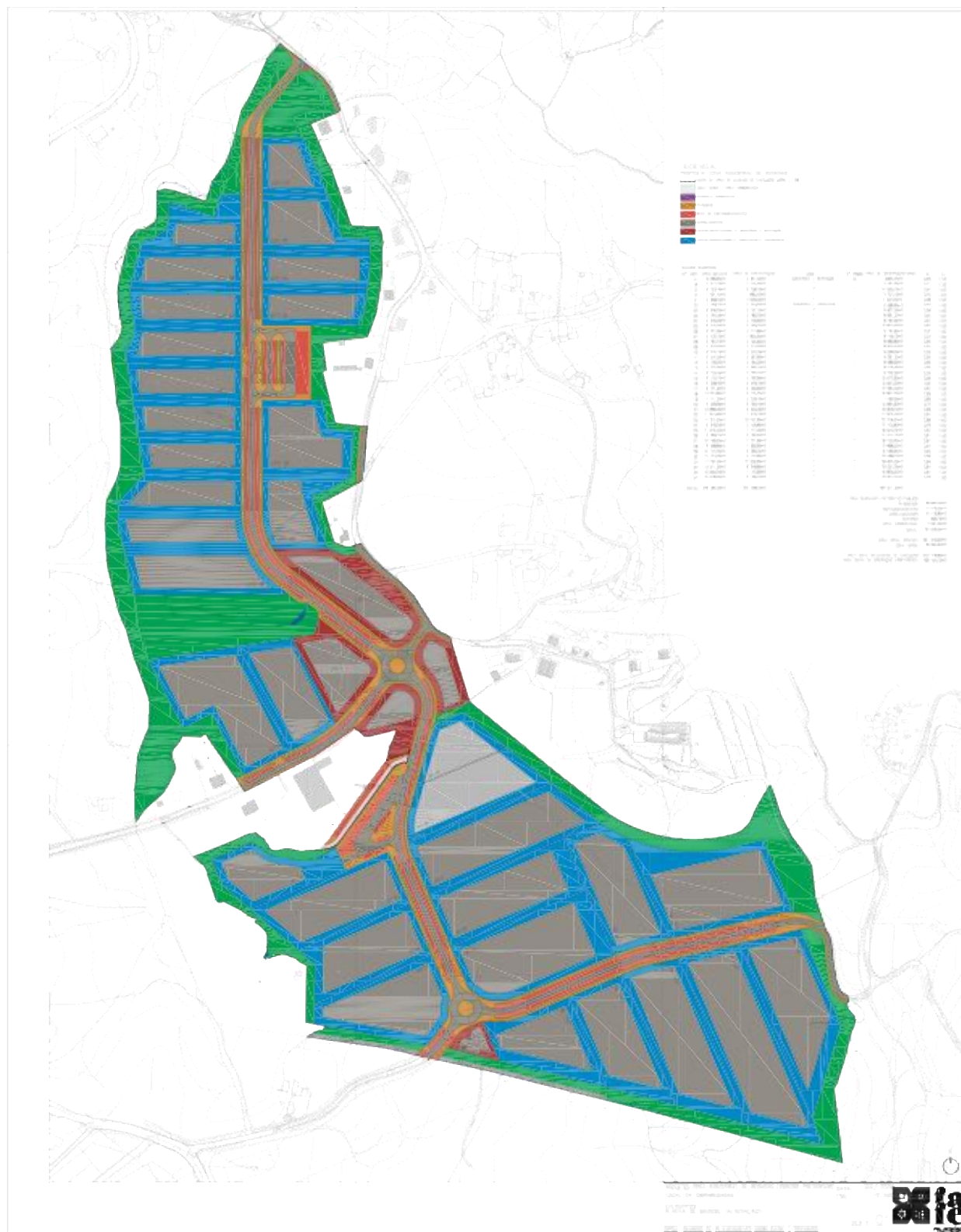
Figura 13 – Planta de Síntese do Loteamento.
