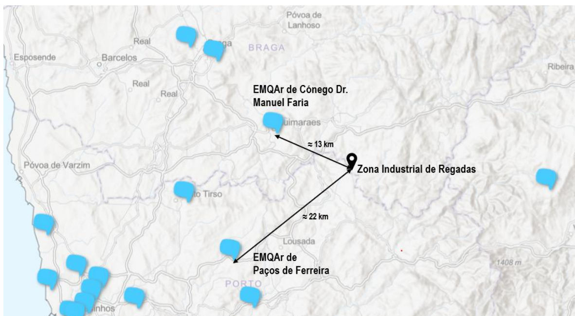
Figura 118 – Localização das estações de monitorização da qualidade do ar mais próximas da área de intervenção.
