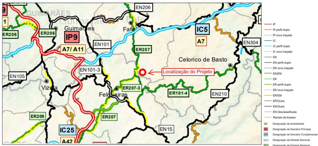
Figura 5 – Mapa da rede rodoviária regional com a área de intervenção.
