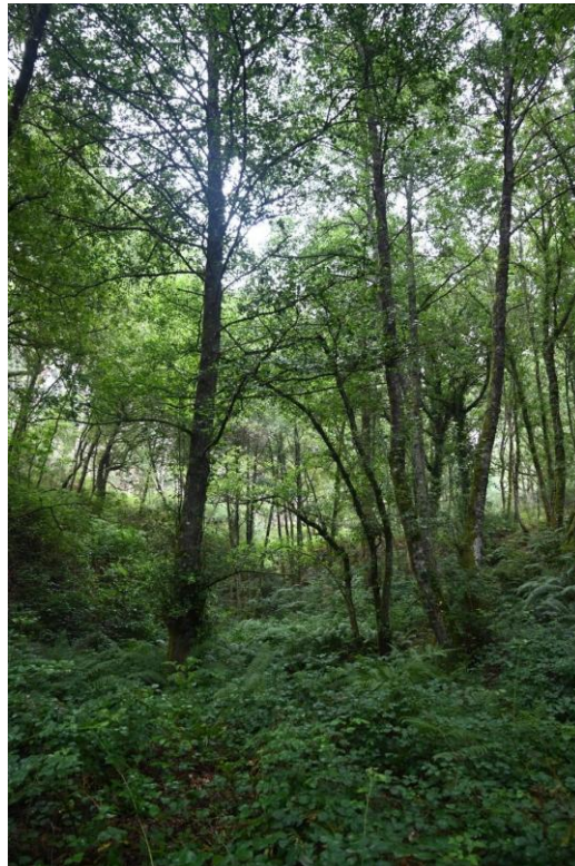
Figura 143 – Localização do inventário 5 em amial ripícola.
