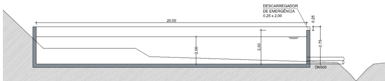
Figura 21 – Corte tipo da bacia de retenção Sul (BR1).
