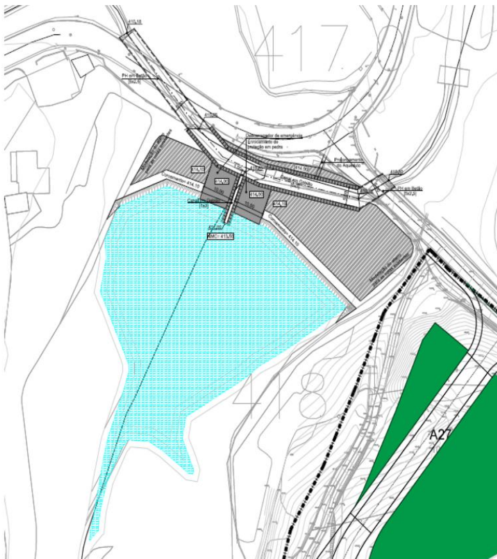
Figura 20 – Planta Bacia de Retenção (BR2), passagens Hidráulicas e Canais.
