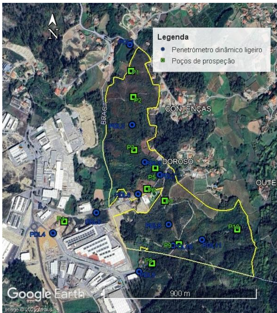
Figura 69 – Pontos de prospeção geotécnica.
