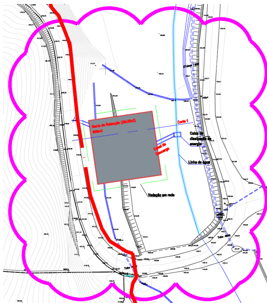
Figura 22 – Planta Bacia de Retenção a sul (BR1).
