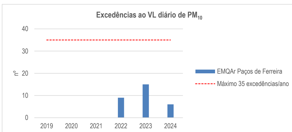
Figura 120 – Dados estatísticos da EMQAr de Paços de Ferreira relativos às excedências ao VL diário de \text{PM}_{10} entre 2019 e 2024.
