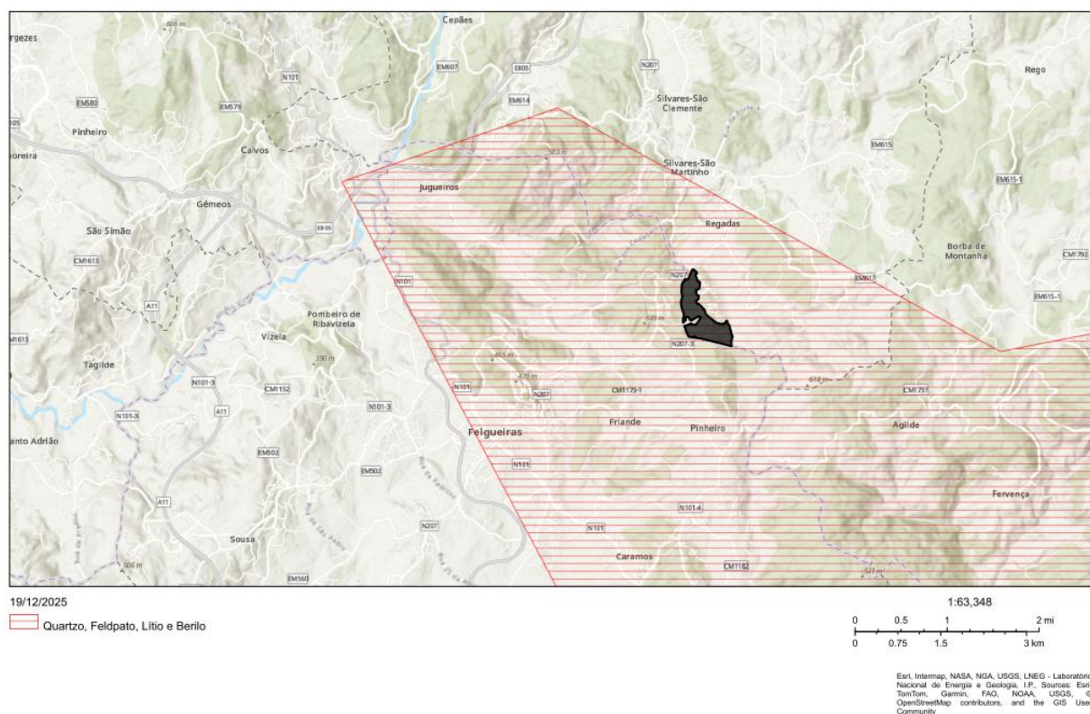
Figura 68 – Projeto sobre áreas potenciais de recursos minerais – (Seixoso-vieiros).
