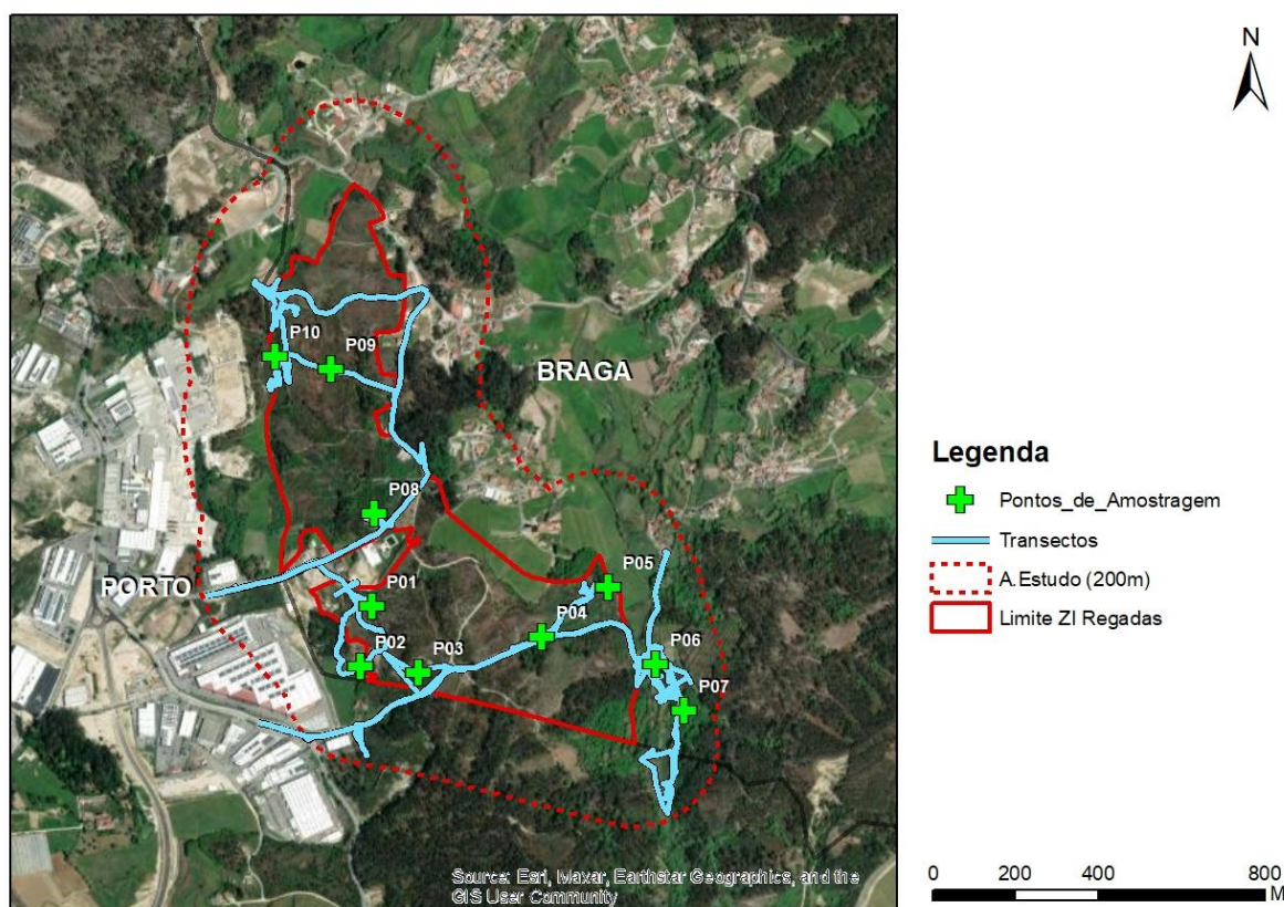
Figura 152 – Locais de amostragem de fauna.
