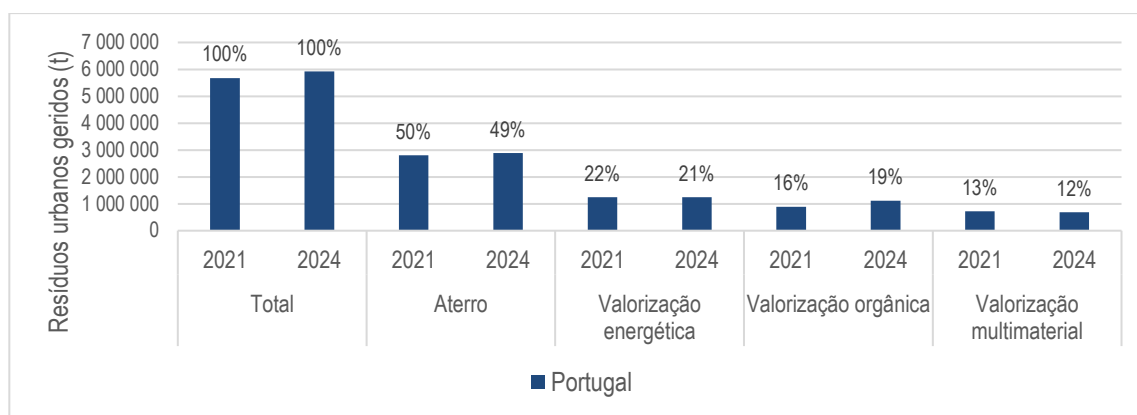
Figura 130 – Resíduos urbanos geridos (t) em Portugal, por tipo de destino (resíduos).
