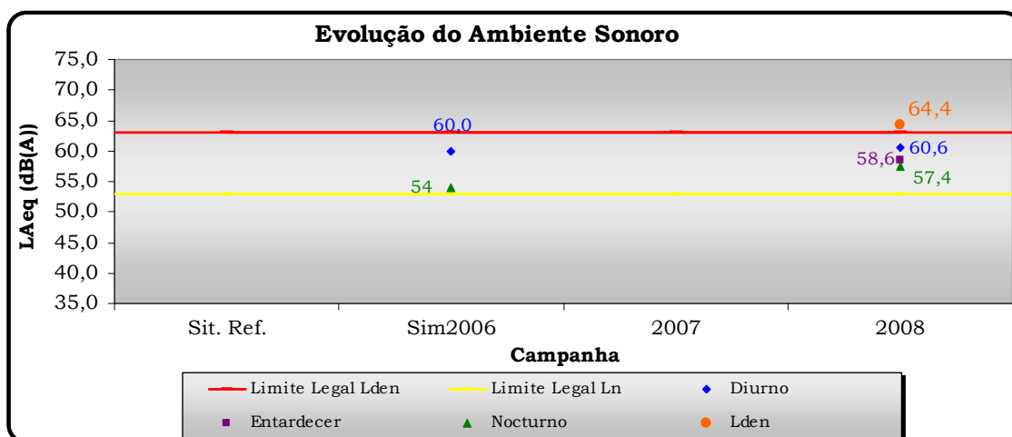
Figura 4.3 – Evolução do ambiente sonoro no ponto P14R.
