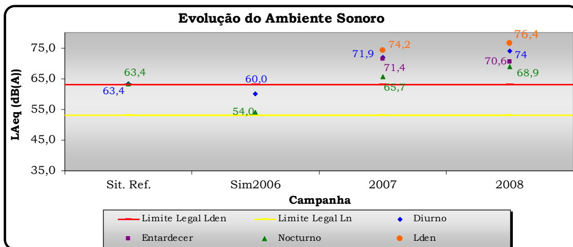
Figura 4.2 – Evolução do ambiente sonoro no ponto P14.
