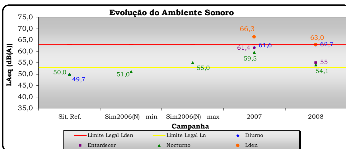
Figura 4.1 – Evolução do ambiente sonoro no ponto P2.
