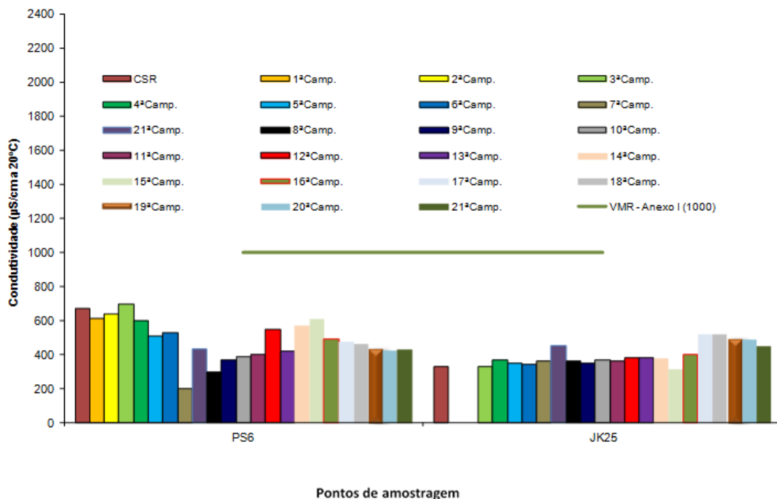
Gráfico 3: Comparação do valor de Condutividade obtido nas campanhas de monitorização
