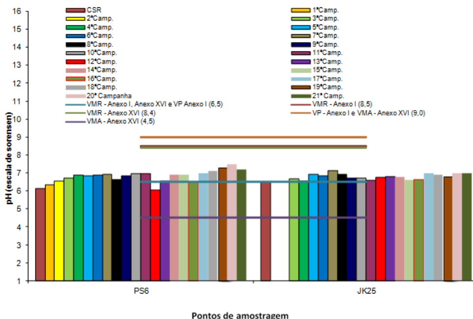
Gráfico 1: Comparação do valor de pH obtido nas campanhas de monitorização
