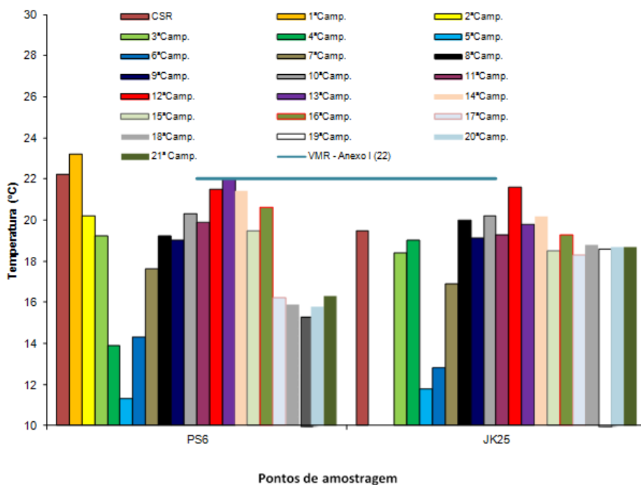
Gráfico 2: Comparação do valor de Temperatura obtido nas campanhas de monitorização
