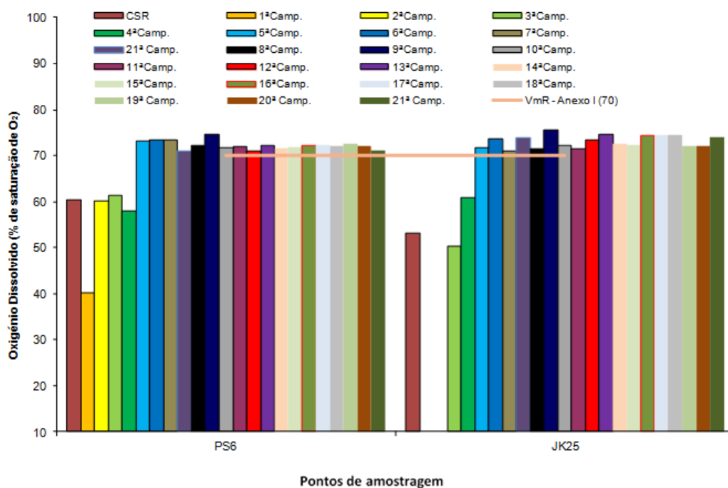
Gráfico 4: Comparação do valor de Oxigénio Dissolvido obtido nas campanhas de monitorização
