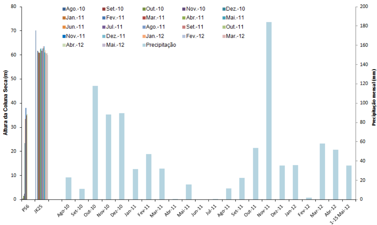
Gráfico 6: Evolução dos valores da Altura de Coluna Seca e Precipitação
