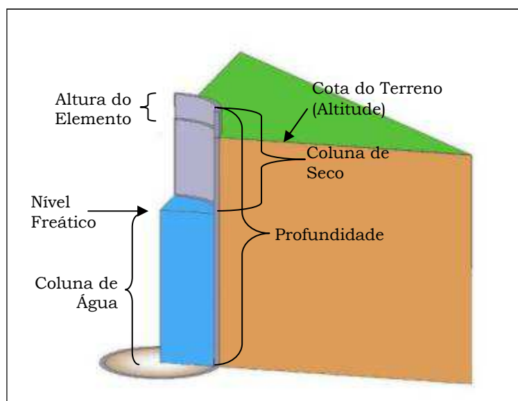
Figura 3.8 – Esquema representativo da metodologia utilizada na medição do nível freático dos poços.
