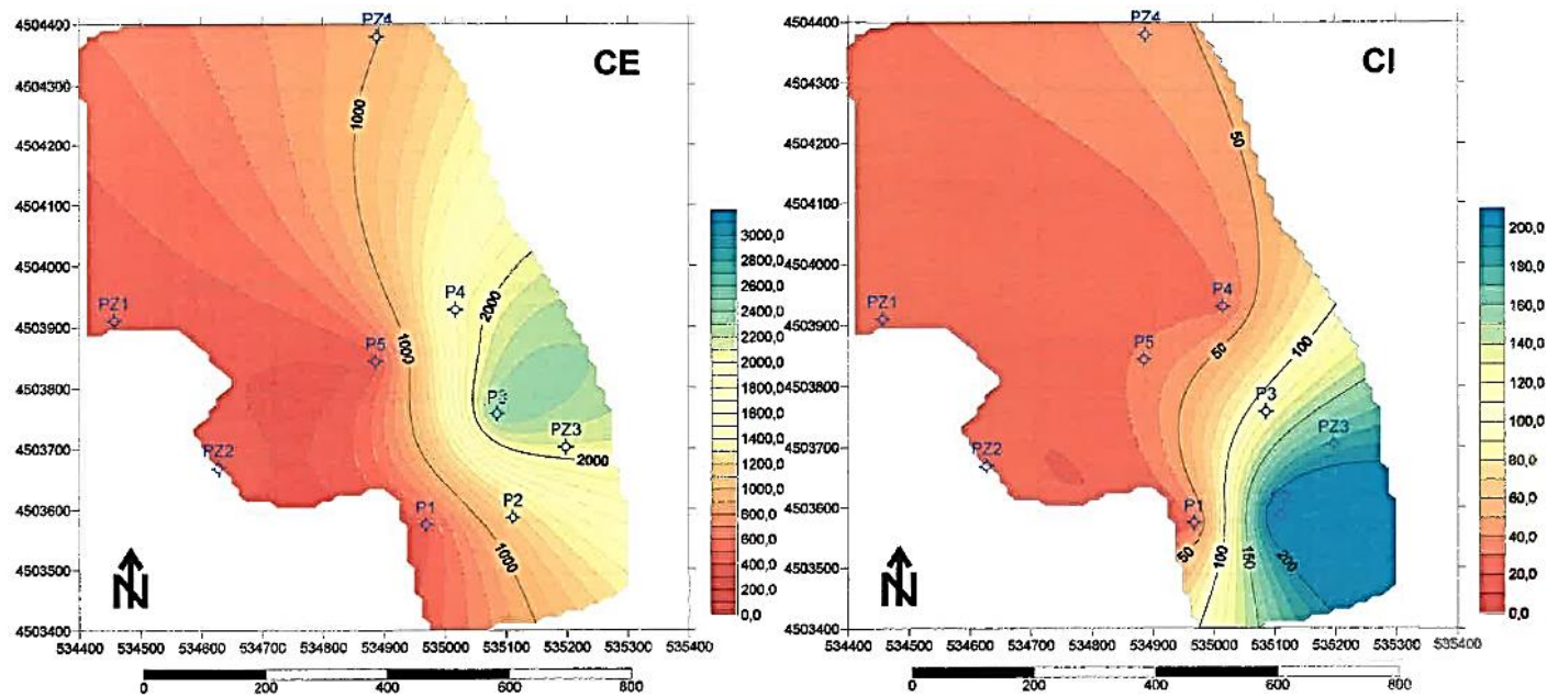
Anexo 9 - Mapa de isovalores de Condutividade Elétrica e Cloretos relativamente ao mês de Maio de 2019.
