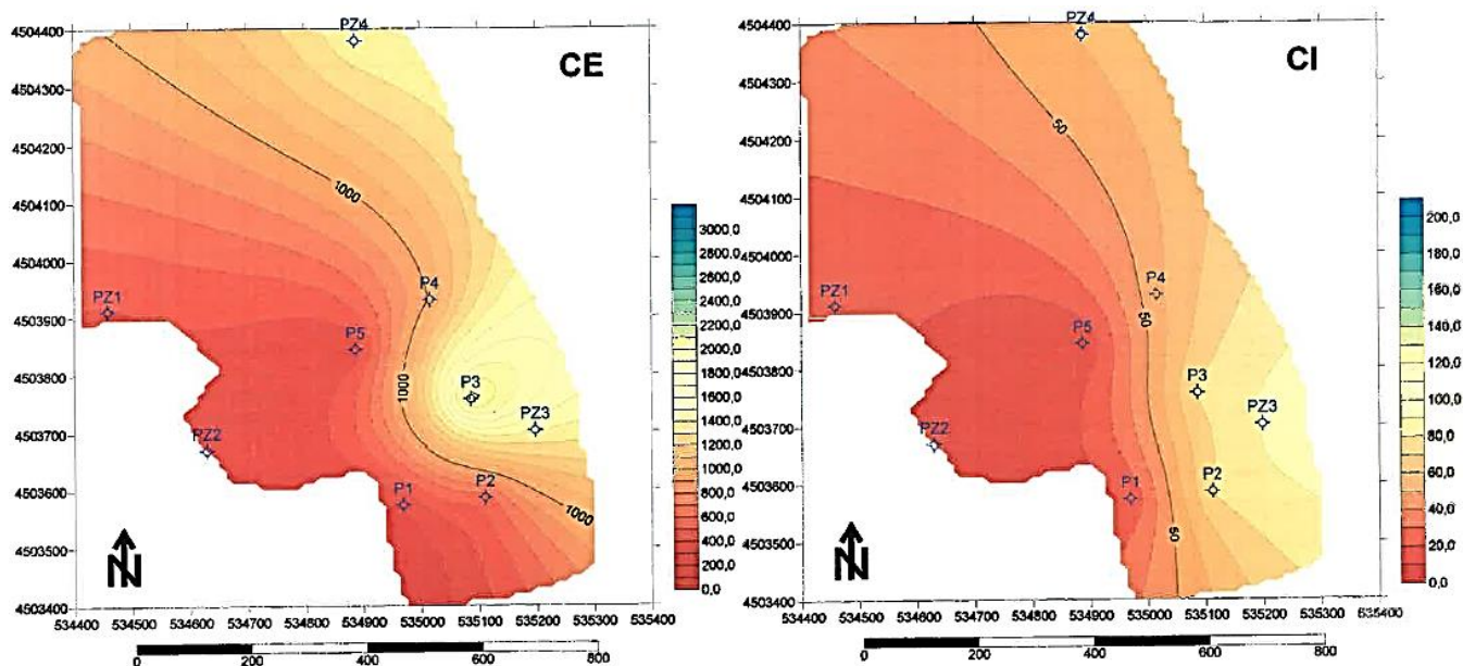
Anexo 21 - Mapa de isovalores de Condutividade Elétrica e Cloretos relativamente ao mês de Novembro de 2019.
