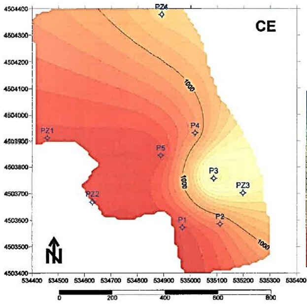
Anexo 17 - Mapa de isovalores de Condutividade Elétrica e Cloretos relativamente ao mês de Setembro de 2019.
