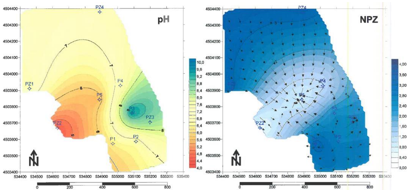
Anexo 4 - Mapa de isovalores de pH e Mapa de isopiezas relativo ao mês de Fevereiro de 2019.
