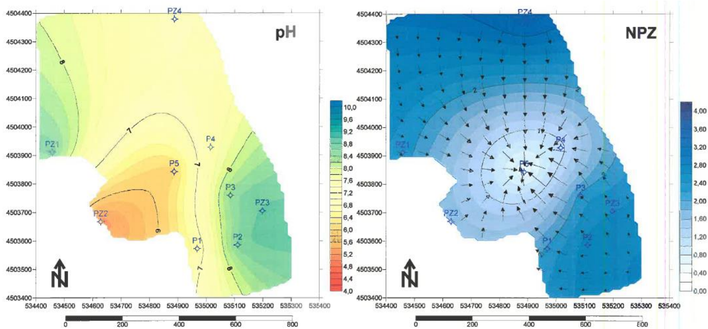
Anexo 12 - Mapa de isovalores de pH e Mapa de isopiezas relativo ao mês de Junho de 2019.
