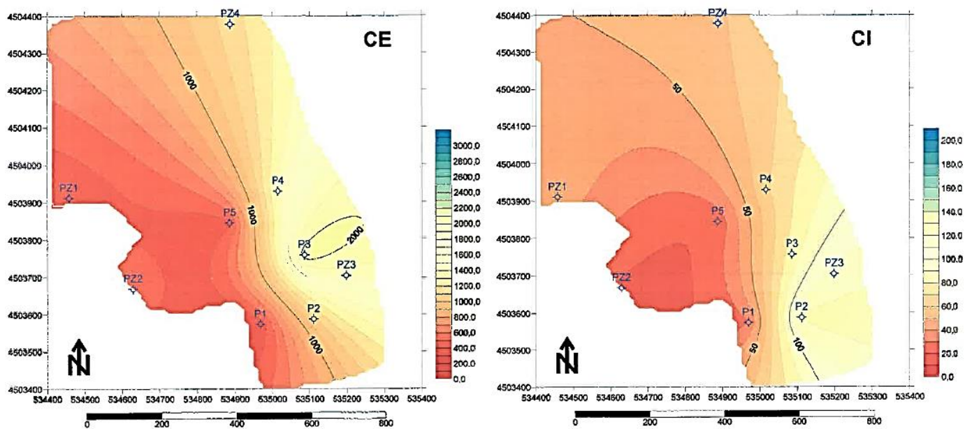
Anexo 15 - Mapa de isovalores de Condutividade Elétrica e Cloratos relativamente ao mês de Agosto de 2019.
