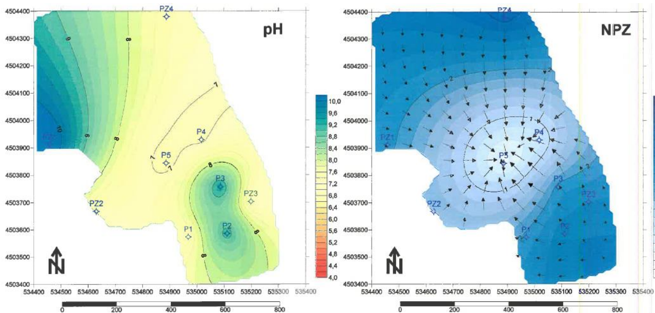
Anexo 6 - Mapa de isovalores de pH e Mapa de isopiezas relativo ao mês de Março de 2019.
