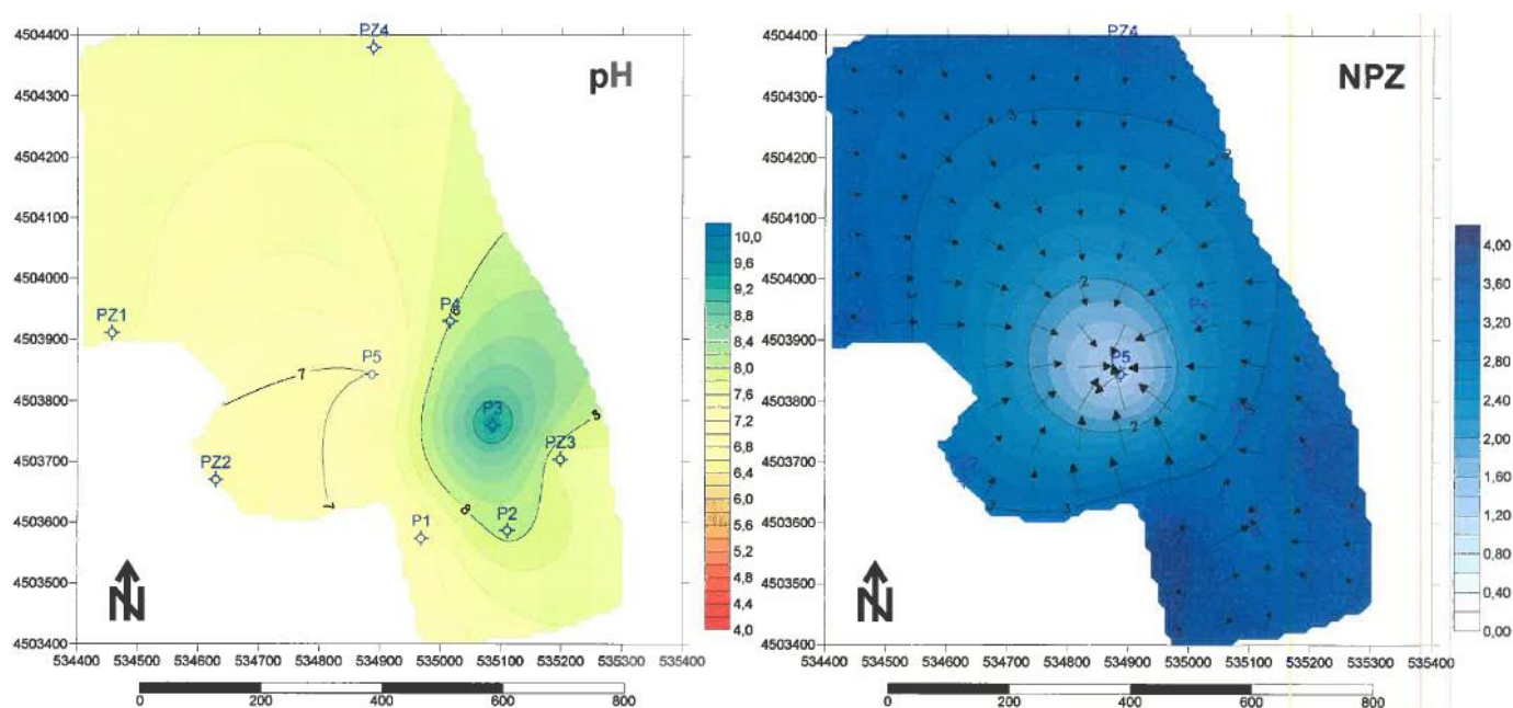
Anexo 24 - Mapa de isovalores de pH e Mapa de isopiezas relativo ao mês de Dezembro de 2019.
