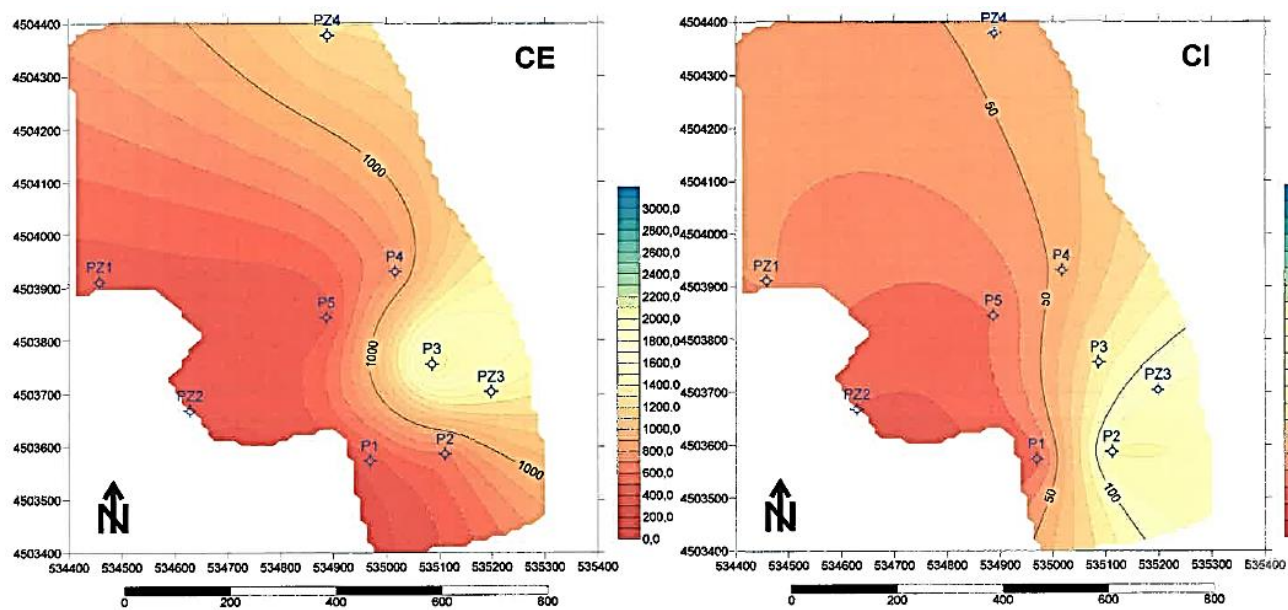
Anexo 19 - Mapa de isovalores de Condutividade Elétrica e Cloretos relativamente ao mês de Outubro de 2019.
