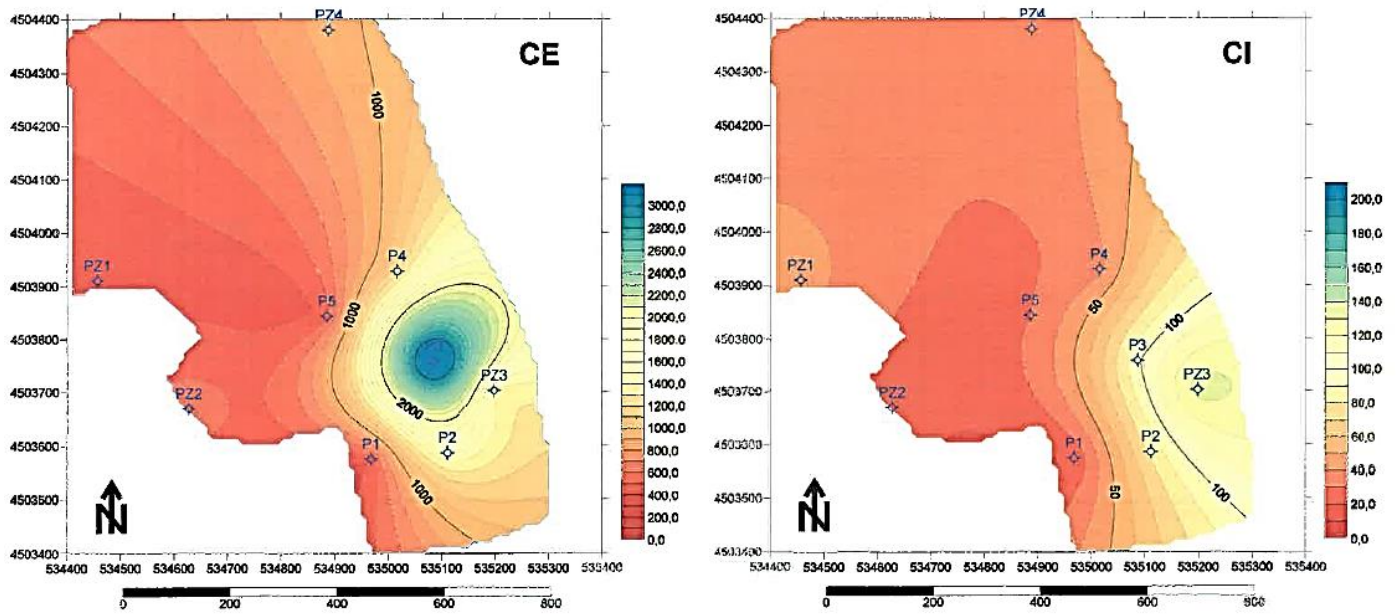
Anexo 5 - Mapa de isovalores de Condutividade Elétrica e Cloretos relativamente ao mês de Março de 2019.
