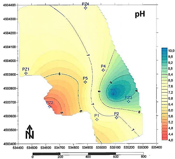
Anexo 2 - Mapa de isovalores de pH relativo ao mês de Janeiro de 2019.
