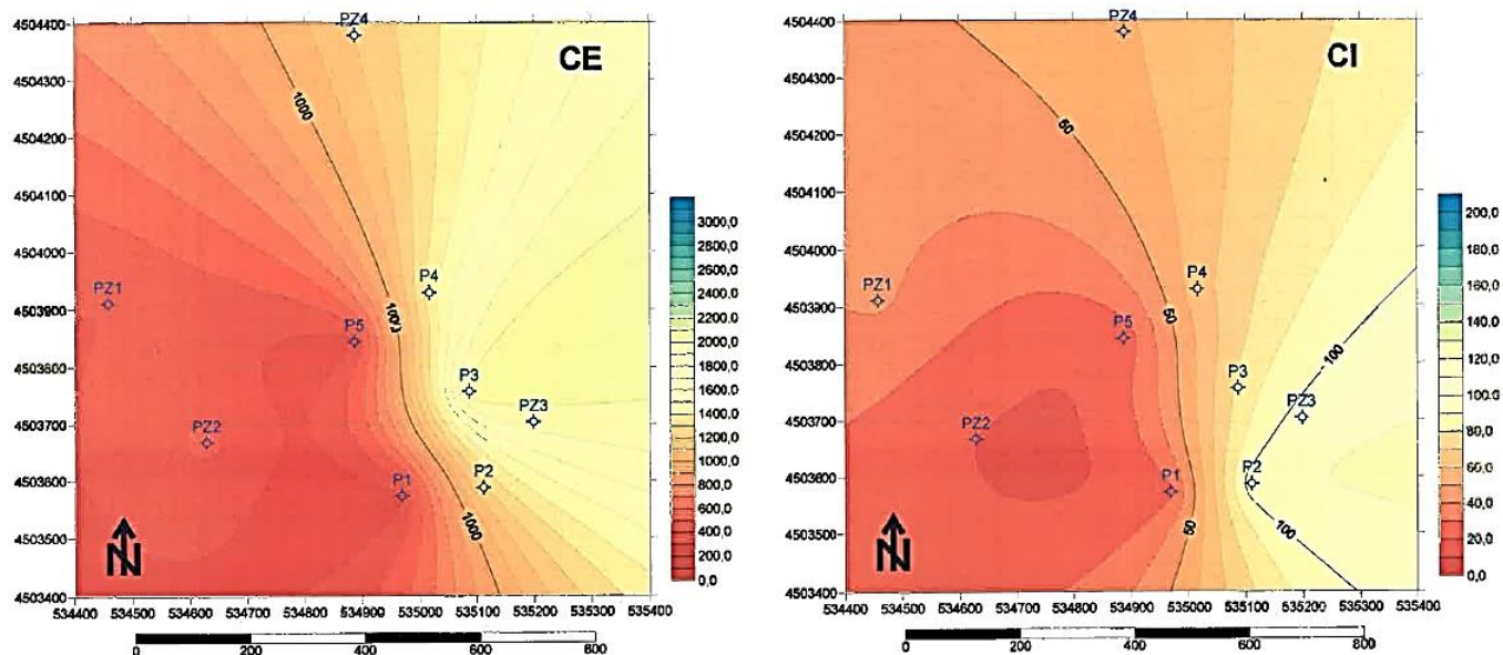
Anexo 13 - Mapa de isovalores de Condutividade Elétrica e Cloretos relativamente ao mês de Julho de 2019.
