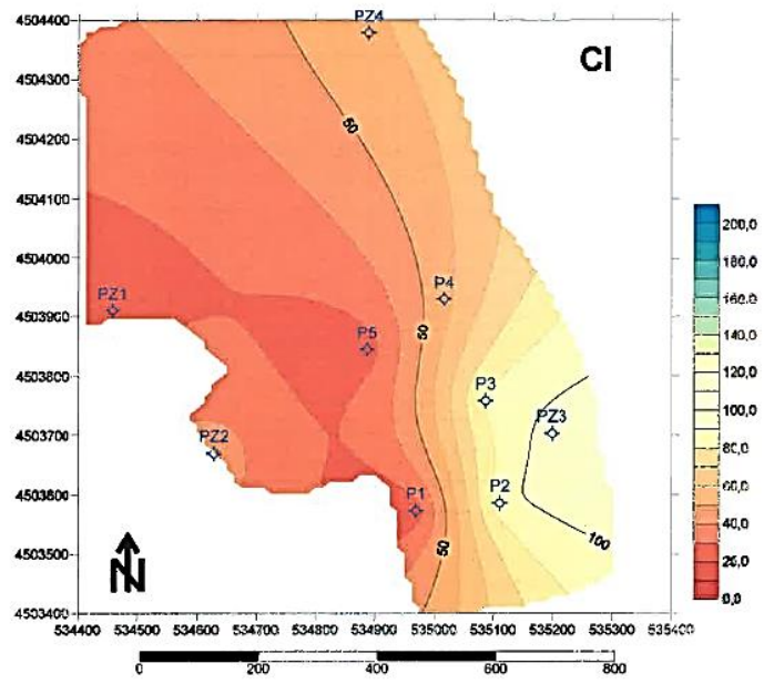
Anexo 17 - Mapa de isovalores de Condutividade Elétrica e Cloretos relativamente ao mês de Setembro de 2019.
