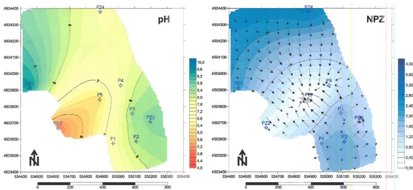
Anexo 16 - Mapa de isovalores de pH e Mapa de isopiezas relativo ao mês de Agosto de 2019.
