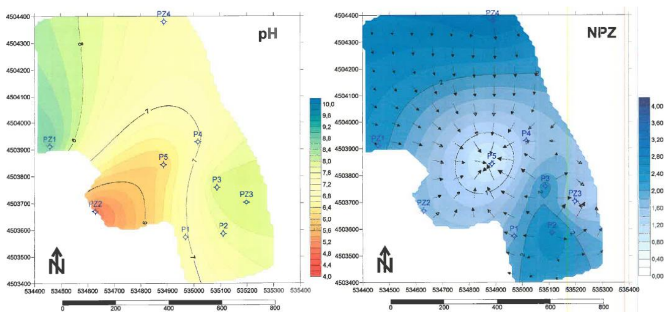
Anexo 22 - Mapa de isovalores de pH e Mapa de isopiezas relativo ao mês de Novembro de 2019.
