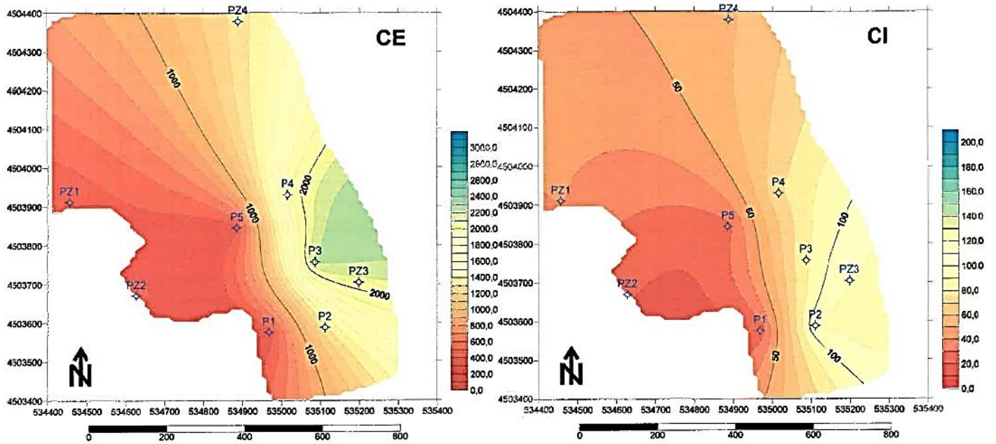
Anexo 11 - Mapa de isovalores de Condutividade Elétrica e Cloretos relativamente ao mês de Junho de 2019.
