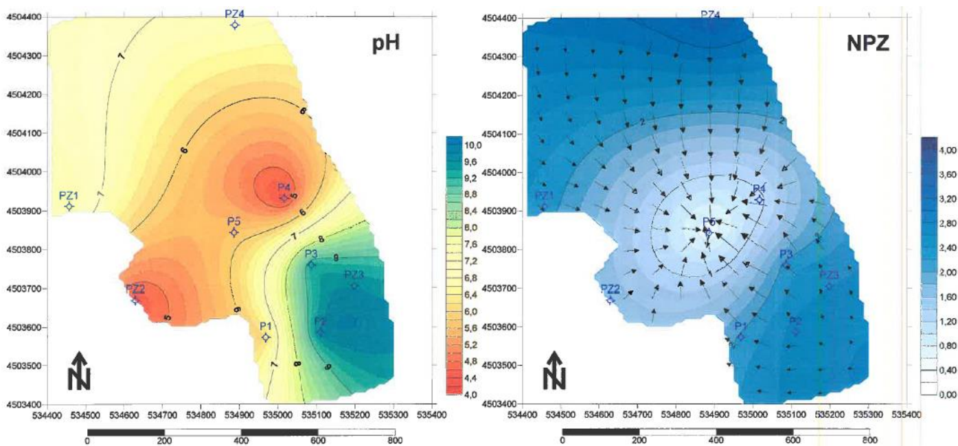
Anexo 8 - Mapa de isovalores de pH e Mapa de isopiezas relativo ao mês de Abril de 2019.
