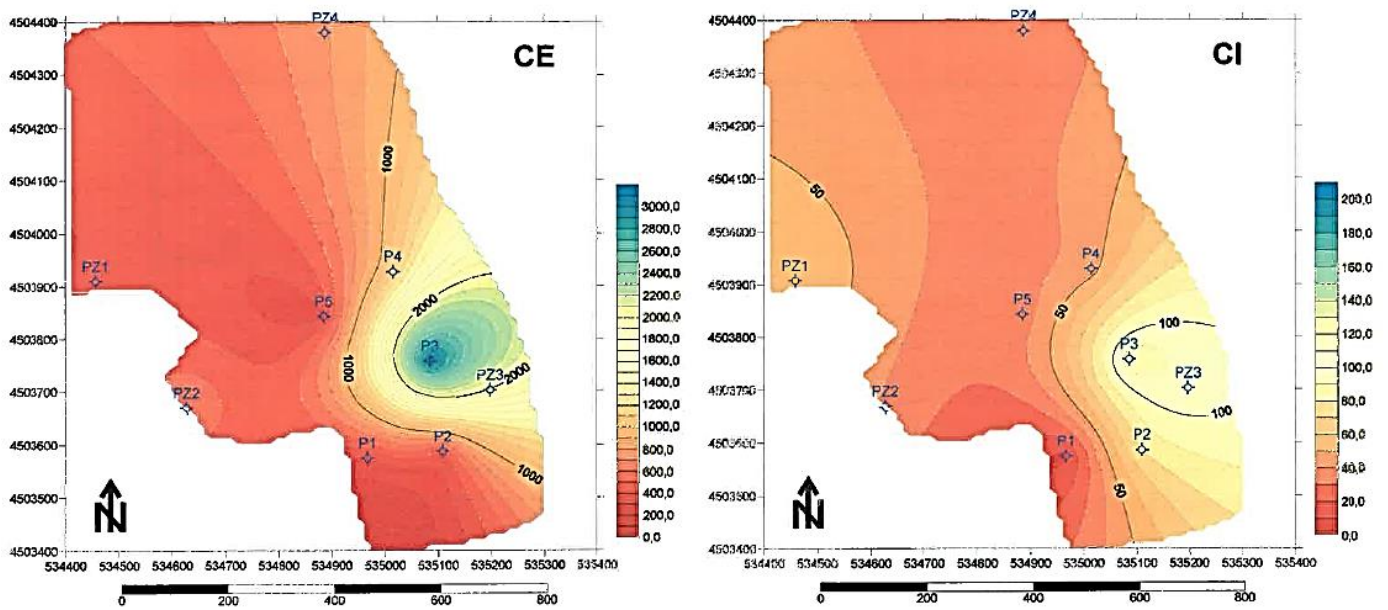
Anexo 3 - Mapa de isovalores de Condutividade Elétrica e Cloretos relativamente ao mês de Fevereiro de 2019.
