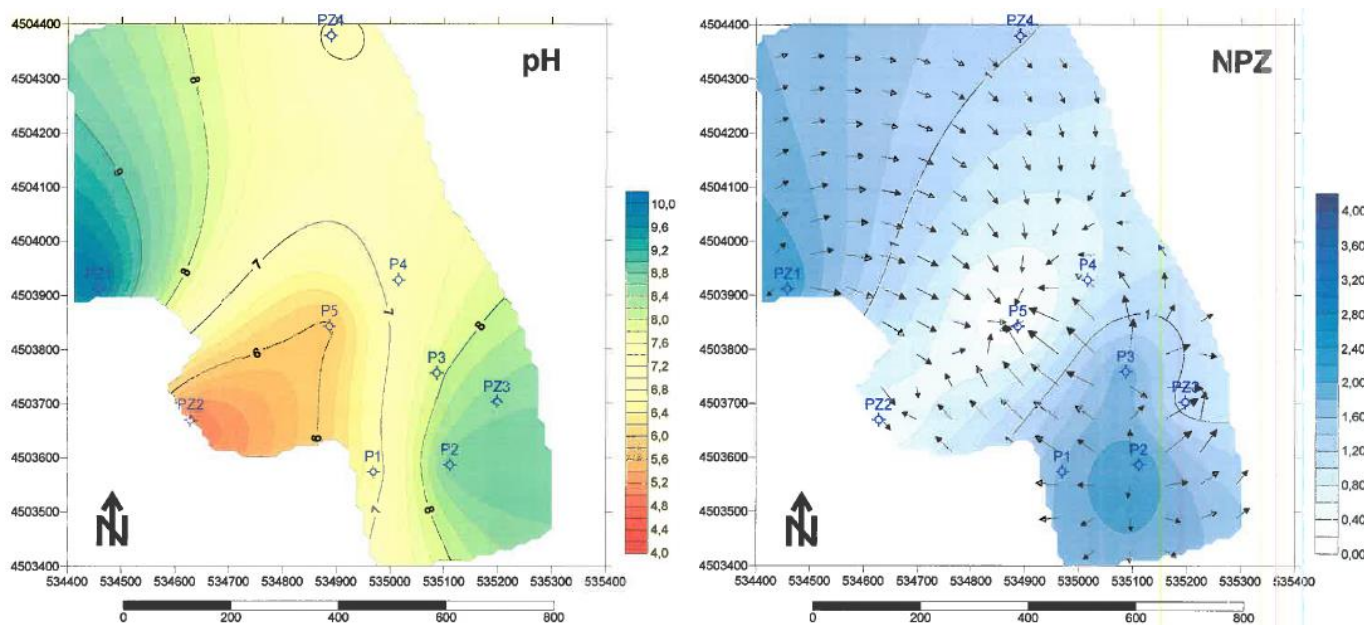
Anexo 14 - Mapa de isovalores de pH e Mapa de isopiezias relativo ao mês de Julho de 2019.
