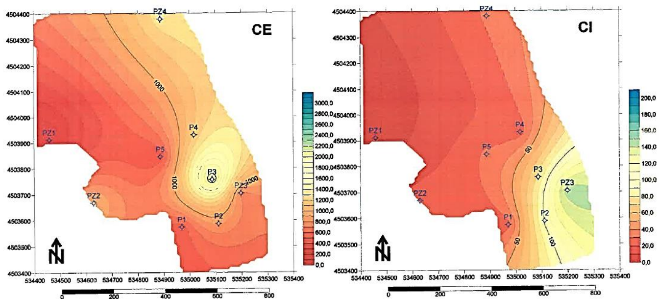
Anexo 23 - Mapa de isovalores de Condutividade Elétrica e Cloretos relativamente ao mês de Dezembro de 2019.
