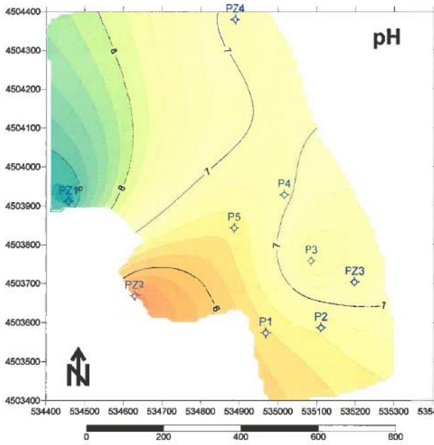
Anexo 18 - Mapa de isovalores de pH e Mapa de isopiezas relativo ao mês de Setembro de 2019.
