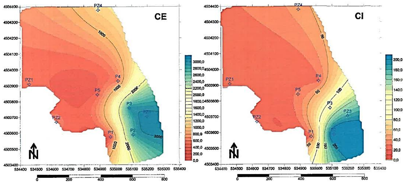
Anexo 7 - Mapa de isovalores de Condutividade Elétrica e Cloretos relativamente ao mês de Abril de 2019.
