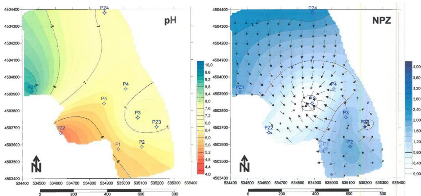
Anexo 20 - Mapa de isovalores de pH e Mapa de isopiezas relativo ao mês de Outubro de 2019.
