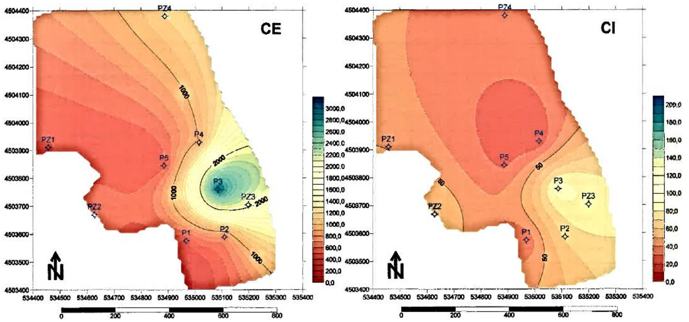
Anexo 1 - Mapa de isovalores de Condutividade Elétrica e Cloretos relativamente ao mês de Janeiro de 2019.
