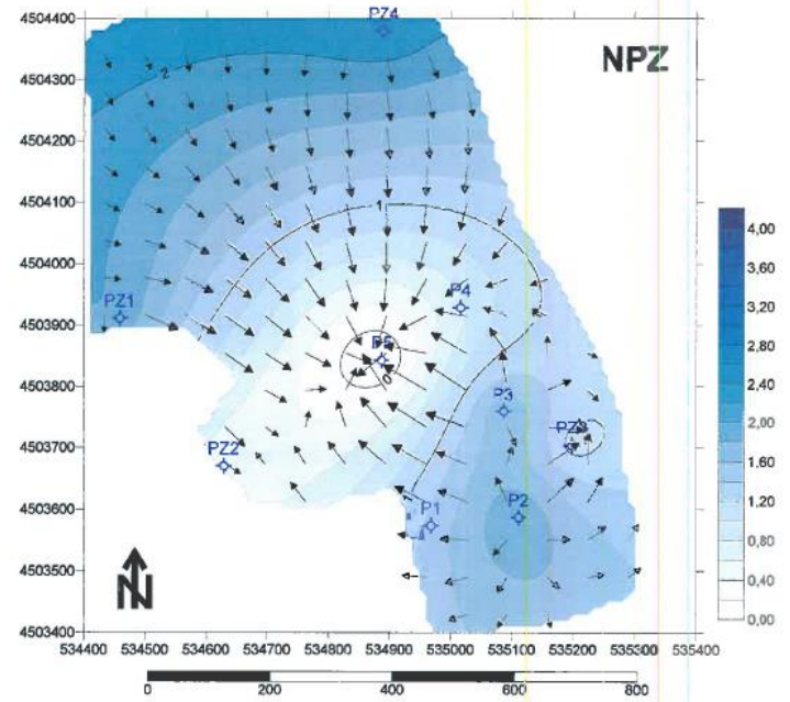
Anexo 18 - Mapa de isovalores de pH e Mapa de isopiezas relativo ao mês de Setembro de 2019.
