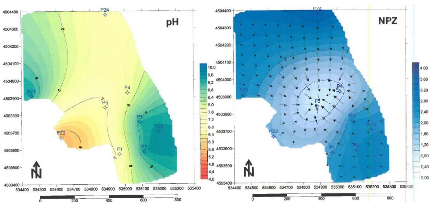
Anexo 10 - Mapa de isovalores de pH e Mapa de isopiezas relativo ao mês de Maio de 2019.
