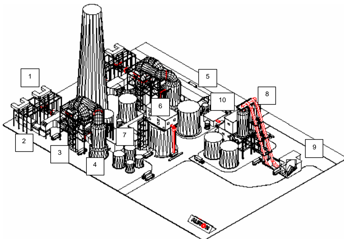
Figura 3 – Central Termoelétrica do Pego com localização dos principais equipamentos da instalação de tratamento de efluentes gasosos.
